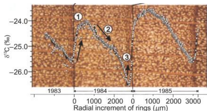
Figure 17. Profil de variation du \delta^{13}\text{C} de la matière organique totale de trois cerne de hêtres ( Fagus sylvatica ) à haute résolution (Helle et al. , 2004)
