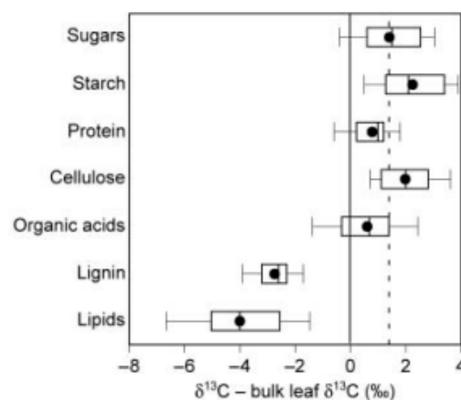
Figure 7. Récapitulatif des compositions isotopiques en carbone de tous les constituants de la feuille d'une plante \text{C}_3 relativement au \delta^{13}\text{C} de la matière organique totale. La ligne correspond au \delta^{13}\text{C} de la matière organique totale de la feuille et la ligne en pointillé indique le \delta^{13}\text{C} des sucres (Bowling et al. , 2008).
