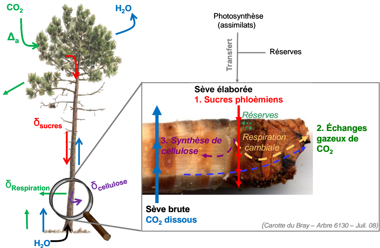
Figure 19. Schématisation des différents flux d'éléments ( \text{CO}_2 et \text{H}_2\text{O} ) et des processus de fonctionnement d'un pin maritime depuis la photosynthèse jusqu'à l'utilisation des sucres phloémiens pour la respiration ou la synthèse de la cellulose déposée dans les cernes annuels.
