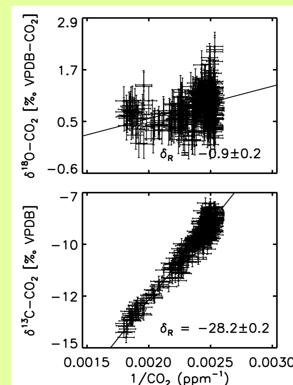
Fig 5: Keeling plot pour \delta^{13}\text{C} et \delta^{18}\text{O} (données de nuit)
