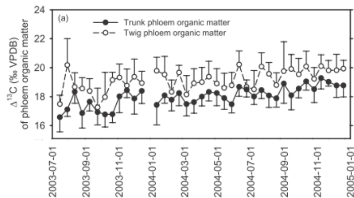
Figure 12. Évolution de la composition isotopique en carbone de la matière organique phloémienne au niveau des rameaux et du tronc d'arbre (Brandes et al. , 2007)
