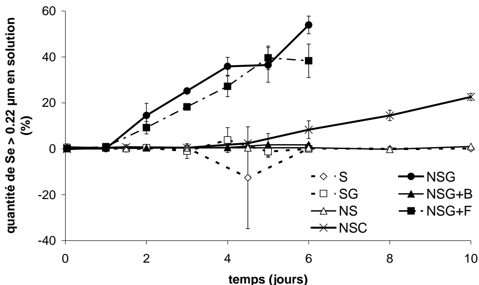
Figure 12: Quantité de Se > 0,22 µm dans le surnageant du batch, exprimée en pourcentage du Se total dans le surnageant. Moyenne des trois réplicats \pm 1 écart-type.
