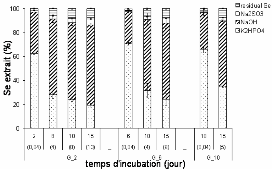
Figure 8: Evolution de la distribution solide du Se. (a) conditions S, C et G (b) conditions G 2 , G 6 et G 10 . Les valeurs entre parenthèses représentent le temps de contact en jour entre le sol et le Se.
