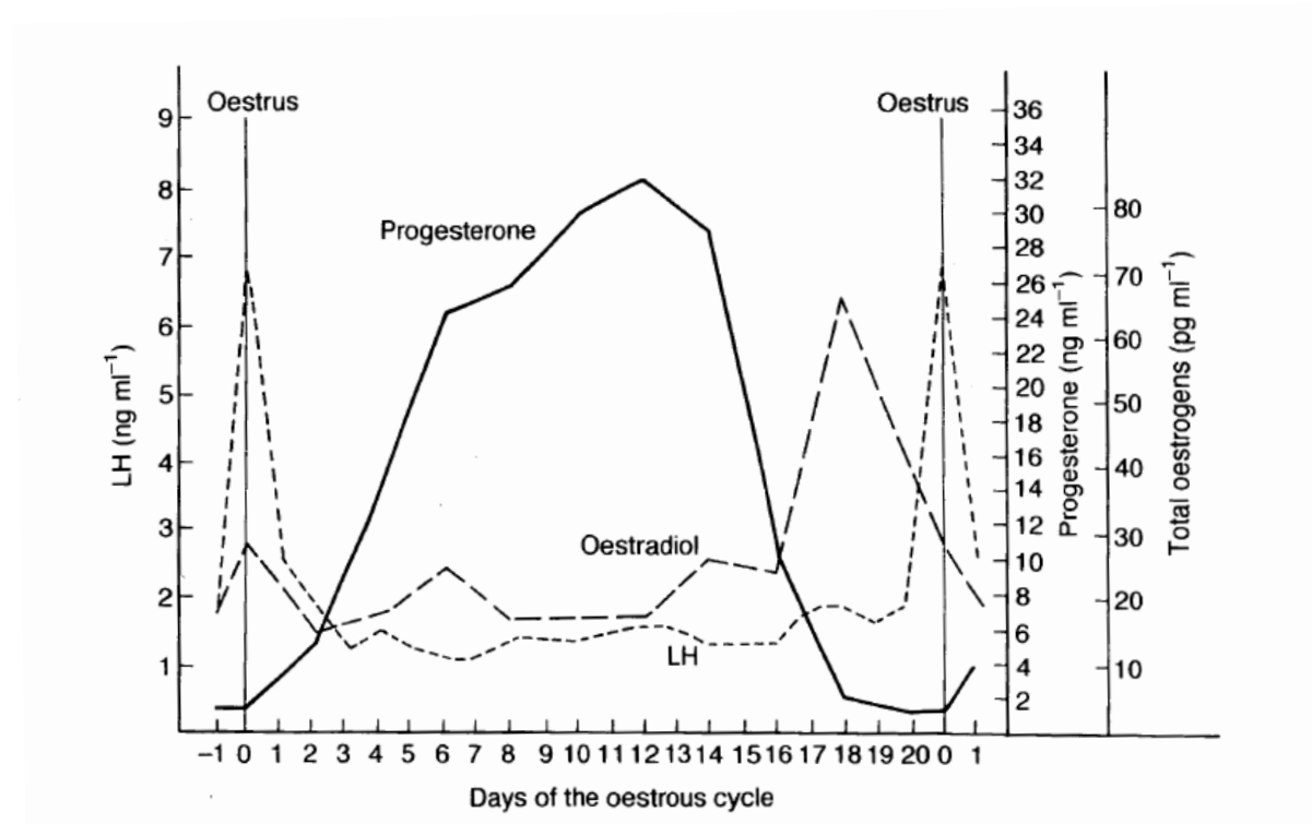
Figure I.1 : Evolution des concentrations en LH, œstradiol et progestérone au cours du cycle sexuel de la truie (d'après Hansel et al. 1973).
