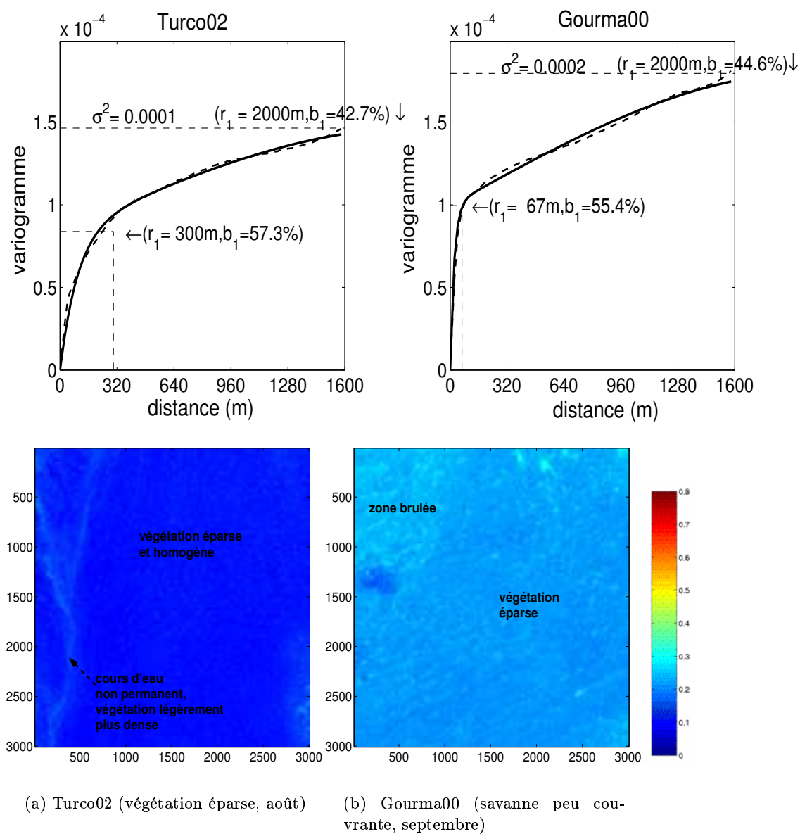
FIG. B.9 – Variogrammes et images du NDVI de Turco02 et Gourma00
