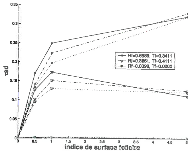
Figure 22 : variation du terme \tau_{sd} , pour \chi=0 , en fonction du LAI [0.5 1 5], ALA [30° (-), 58°(--), 70°(....)] et les propriétés optiques des feuilles. Les autres caractéristiques sont identiques à celles de la Figure 19.
