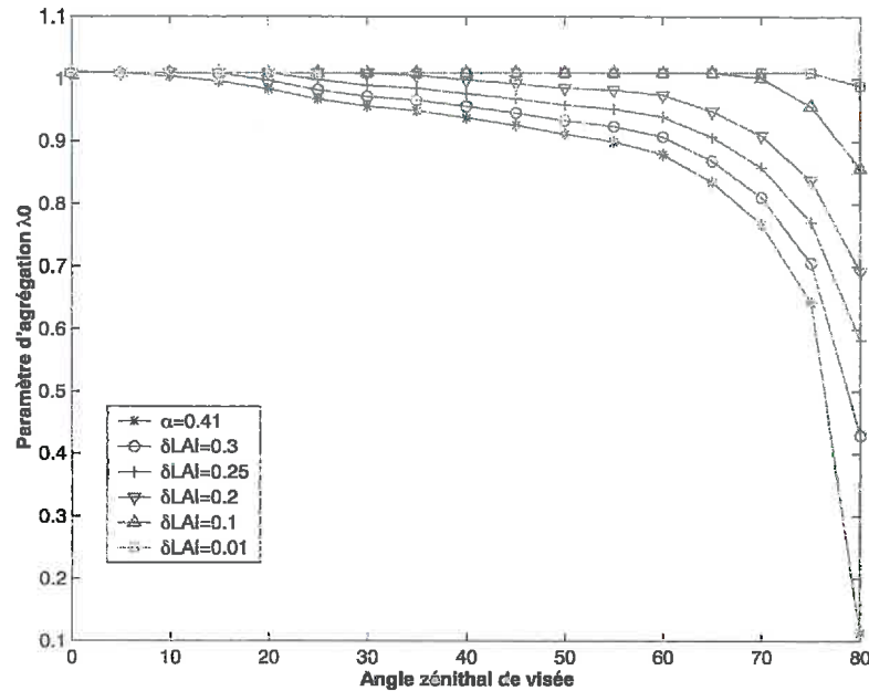
Figure 7 : Sensibilité du paramètre d'agrégation \lambda à l'épaisseur de la couche pour toutes les directions zénithales. La maquette décrit un milieu aléatoire avec \chi=1 , S^*=1 , d^*=1 , b/h=0.25 et pour un LAI= 1
