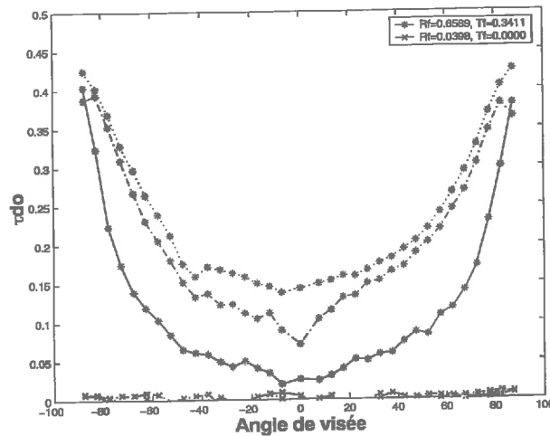
Figure 28 : variation du terme \tau_{do} en fonction de l'angle de visée dans le plan principal, d^* [1(-) 10(--), 100(...)], \chi=0 , et propriétés optique des feuilles. Les autres caractéristiques sont identiques à celles de la Figure 19.
