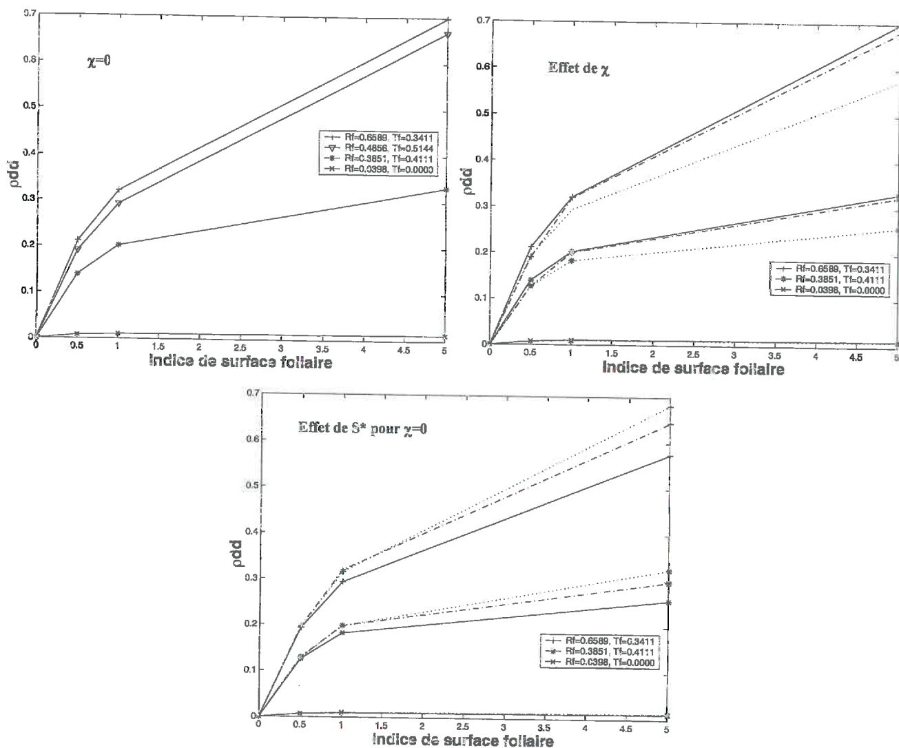
Figure 23 : variation du terme \rho_{dd} en fonction du LAI [0.5 1 5], S^* [0.025 (-), 0.05(-), 0.1(...)], \chi =[0(...), 0.5(--), 1(-)], et les propriétés optique des feuilles. Les autres caractéristiques sont identiques à celles de la Figure 19
