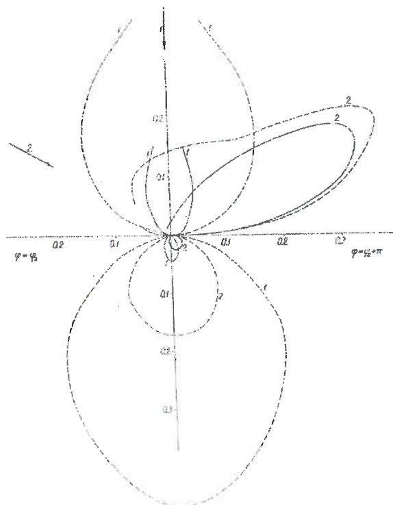
Figure 2 : distribution angulaire du rayonnement diffusé par unité de surface d'une feuille de maïs dans le bleu (trait plein).et le proche infrarouge (pointillé) pour deux angles d'incidence 0^\circ (1) et 60^\circ (2) (Ross 1981).
