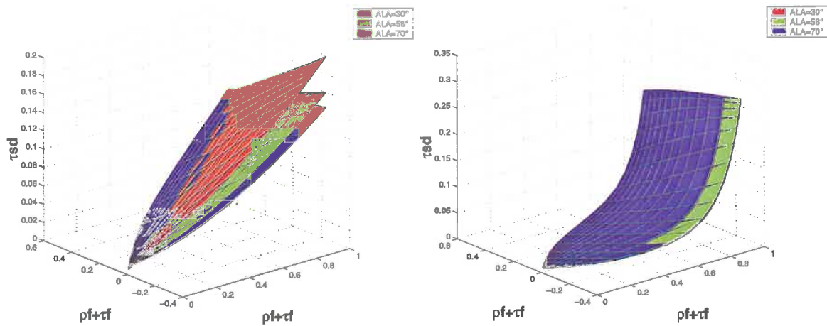
Figure 8 : idem Figure 6 mais pour différents angles moyens d'inclinaisons. ALA=[30°, 58°, 70°] et LAI=0.5 (à gauche) ou 7 (à droite).
