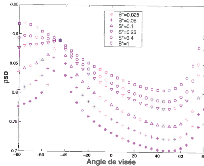
Figure 16 : variation directionnelle dans le plan principal de la réflectance directionnelle-directionnelle en fonction de la taille de la feuille. LAI=7^\circ ; ALA=30^\circ ; \rho_f=0.38 \tau_f=0.62 .
