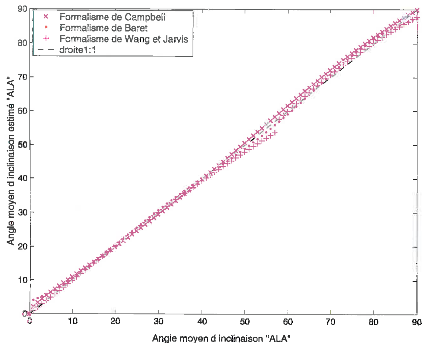
Figure 4 : Comparaison des angles d'inclinaison moyen estimés à partir de deux expressions semi-empiriques différentes du rapport de l'axe horizontal sur l'axe vertical de l'ellipsoïde ' \delta ' dans le cas d'une distribution ellipsoïdale
