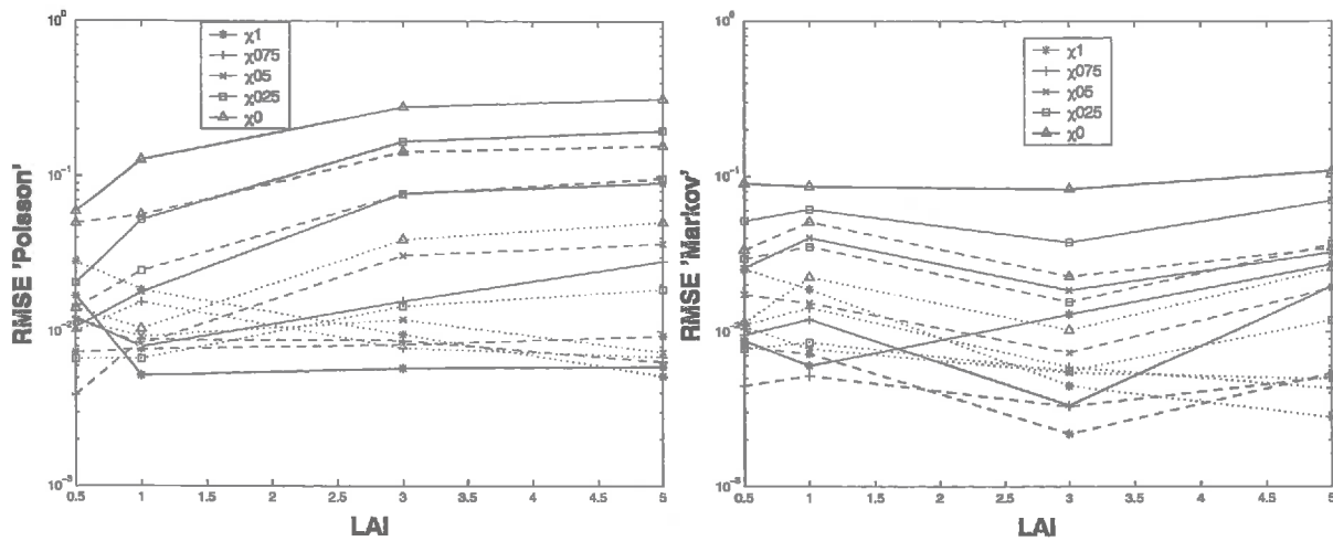
Figure 12 : Exemple de sensibilité à l'indice foliaire de l'erreur quadratique moyenne des deux modèles pour \chi=[0.25 \ 0.5 \ 0.75 \ 1] , S^*=[0.025 \ \dots; 0.05 \ \dots, 0.1 \ \dots] , d^*=100pt , b/h=0.25 , ALA=58^\circ .
