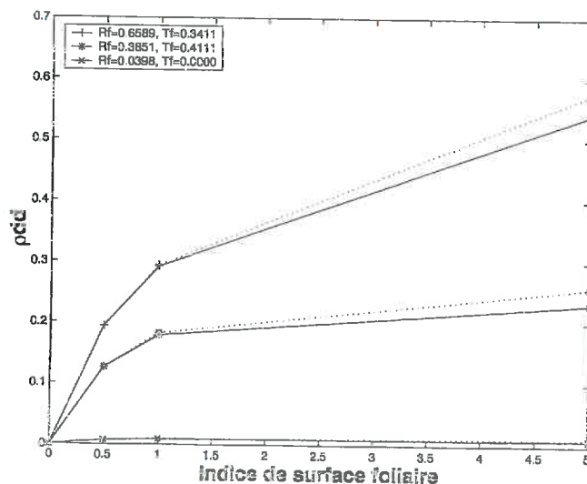
Figure 24 : variation du terme \rho_{dd} en fonction du LAI [0.5 1 5], b/h [0.25 (-), 1(--)], \chi =0, et les propriétés optique des feuilles. Les autres caractéristiques sont identiques à celles de la Figure 19
