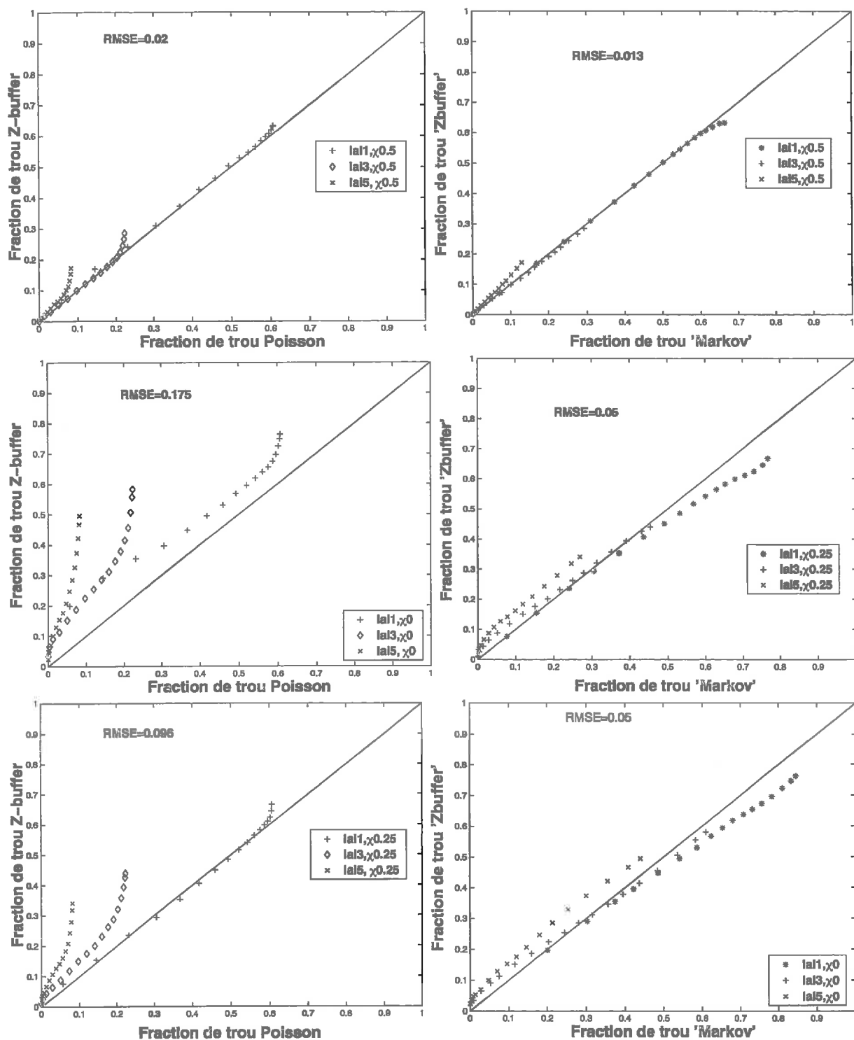
j Figure 10 Comparaison de la fraction de trous mesurée par Z-buffer pour tous les angles de visées aux simulations des modèles de Poisson et Markov. Les maquettes considérées décrivent des milieux agrégés avec \chi = [0, 0.25, 0.5] , LAI=[1 3 5], d^*=10 , S^*=0.1 , ALA=58° et b/h=0.25.
