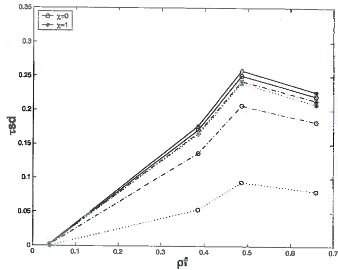
Figure 21 : variation du coefficient \tau_{sd} en fonction de la densité des plantes, d^* [1(...), 10(--), 100(-)], et la réflectance des feuilles : LAI=1, S^*=0.1 , ALA=58°. Les autres caractéristiques sont identiques à celles de la Figure 19.
