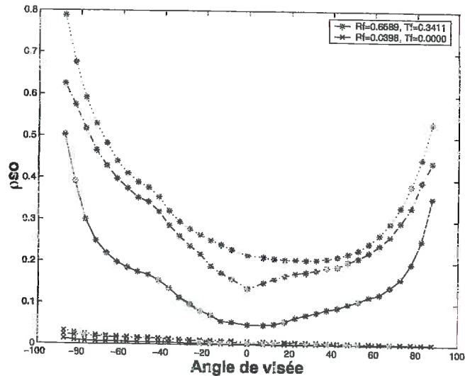
Figure 32 variation du terme \rho_{so} en fonction de l'angle de visée dans le plan principal, d^* [1(-) 10(-- ) 100(...)], \chi=0 , et propriétés optique des feuilles Les autres caractéristiques sont identiques à celles de la Figure 19.
