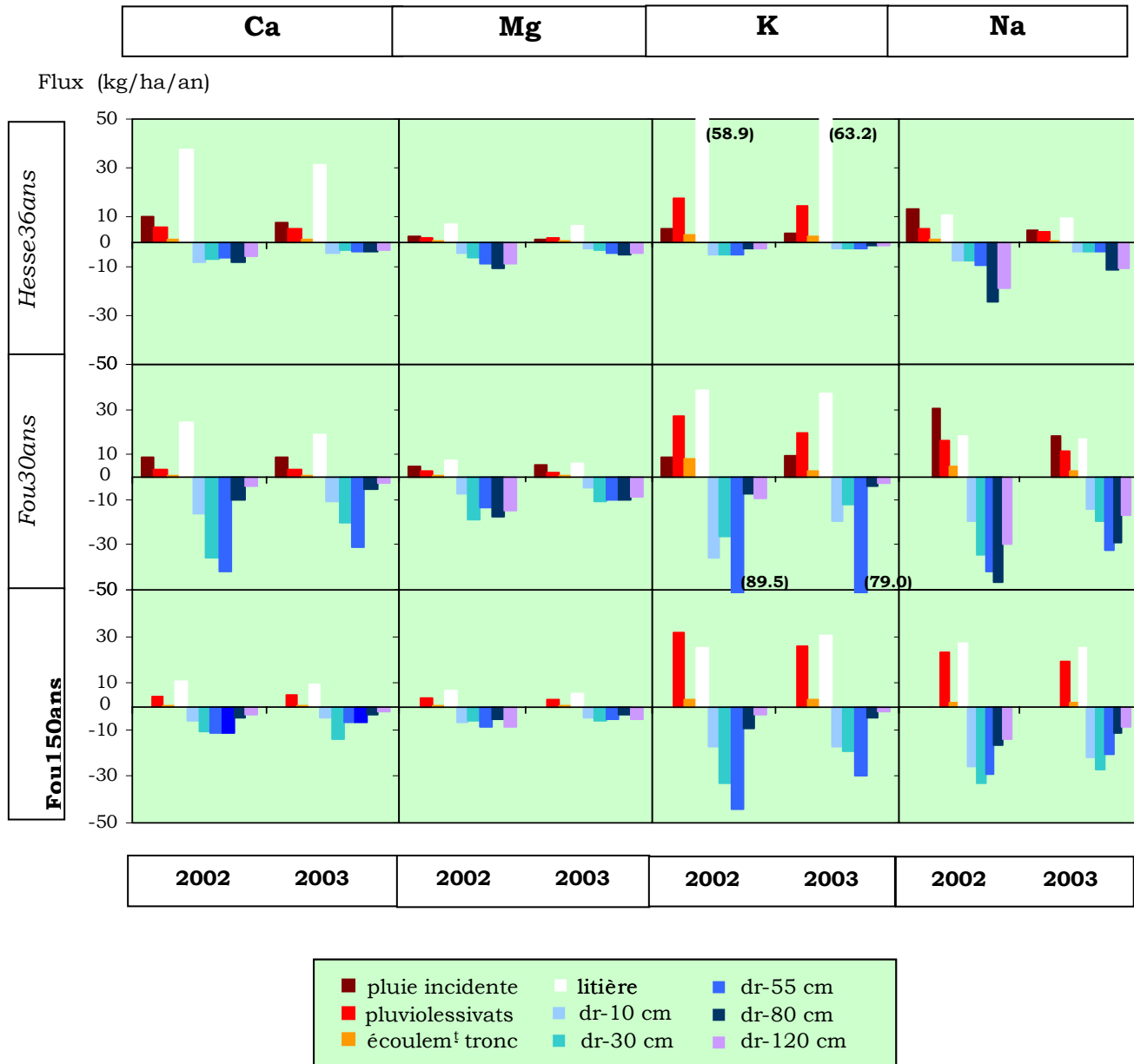
Figure 57 : Comparaison des flux annuels de Ca, Mg, K et Na en 2002 et 2003 (en kg/ha/an). Les entrées dans le sol par les pluies incidentes, pluviolessivats, écoulements le long des troncs et litière sont représentées en positif et les sorties par drainage à 10, 30, 55, 80 et 120 cm de profondeur sont représentées en négatif.
