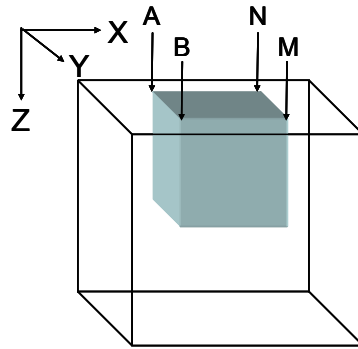
Figure IV-9 : Schéma synthétique du volume prospecté par un dispositif carré ABMN, centré par rapport à X et Y dans un milieu homogène.
