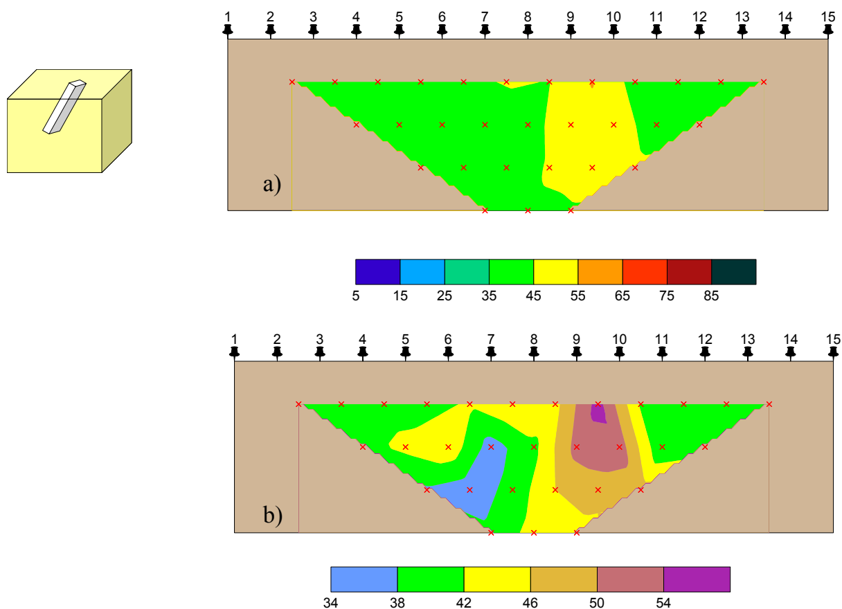
Figure III-18 : Répartition des résistivités apparentes pour une fissure de 0,004 m de large et 0,030 m de profondeur entre les électrodes 9 et 10 orientée à 45° vers la gauche, a) échelle identique aux autres cartes de résistivité, b) échelle réduite.
