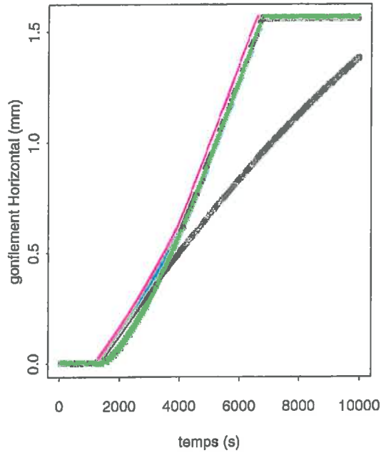
d : gonflement horizontal à 70 cm,
