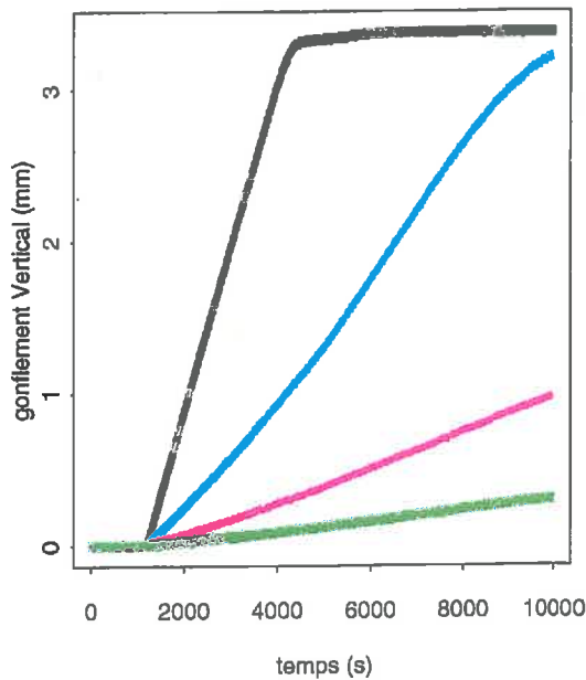
b : couche 30 - 50 cm
