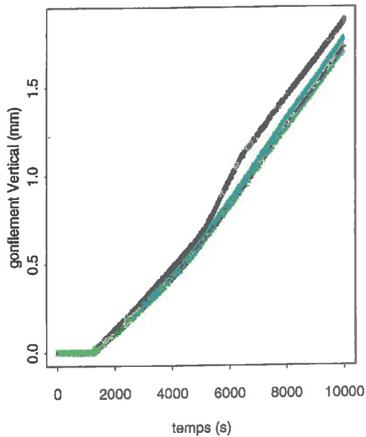
c : couche 50 - 70 cm
