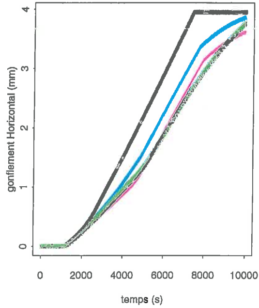
b : gonflement horizontal à 30 cm,
