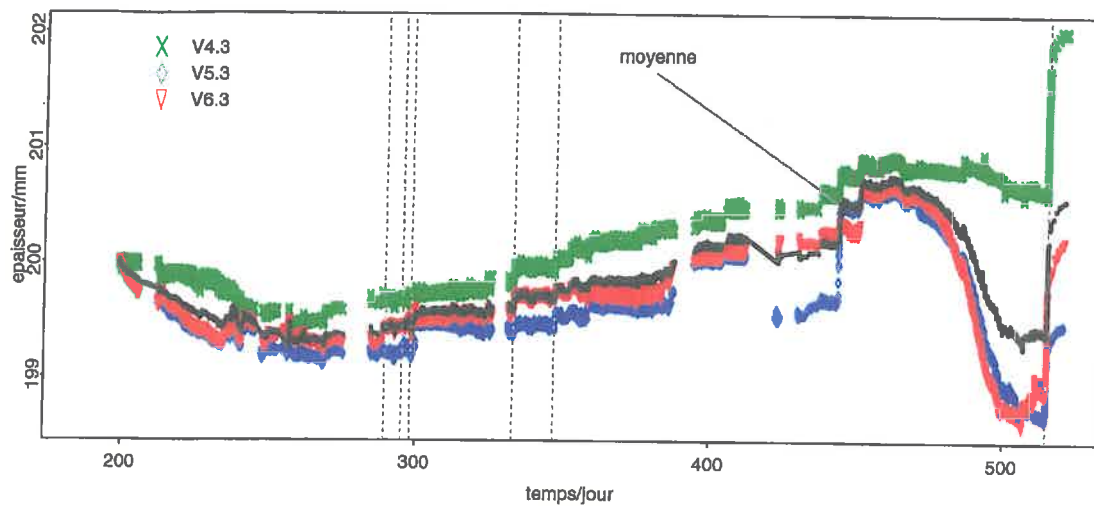
Graphe VIII-14 : variations d'épaisseur de la couche 70-90 cm, Gardel - INRA.
