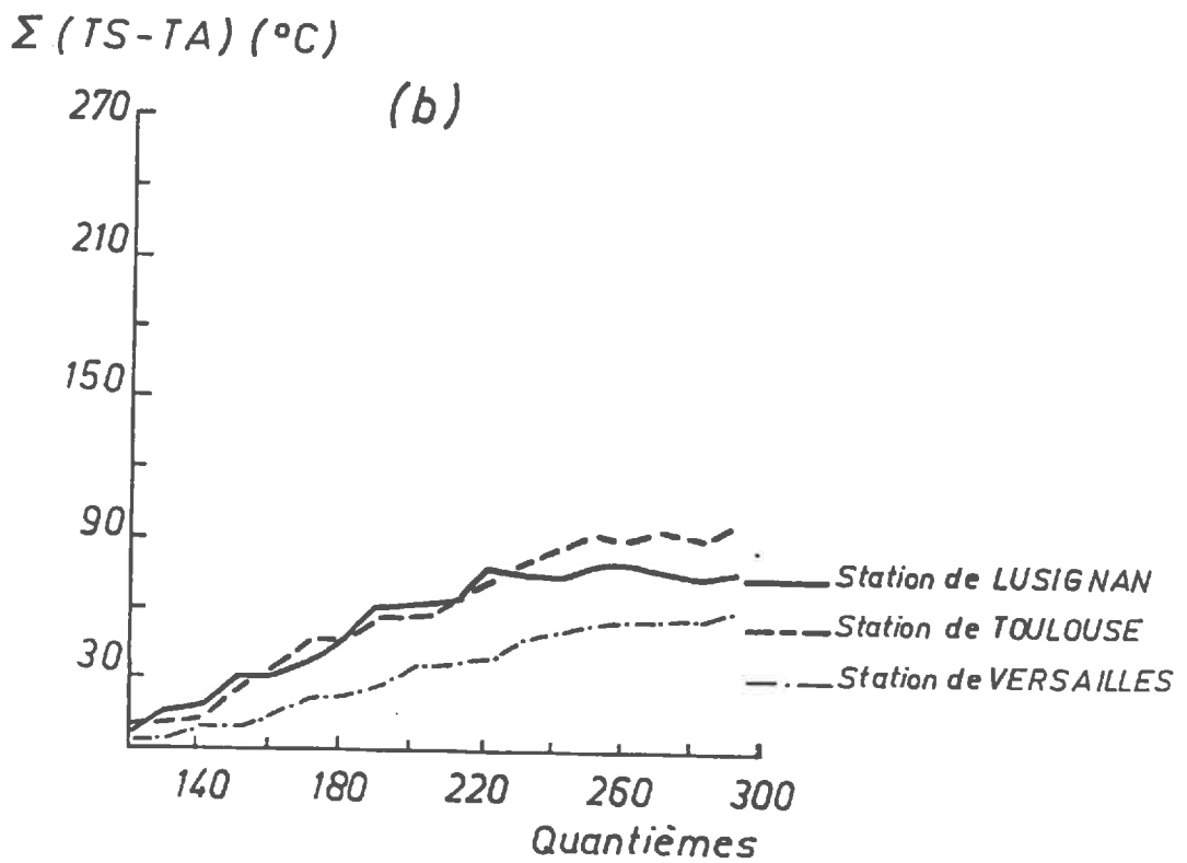
FIGURE IV.15: Classifications climatiques des stations en fonction des valeurs de Stress Degree Day : 1987.
