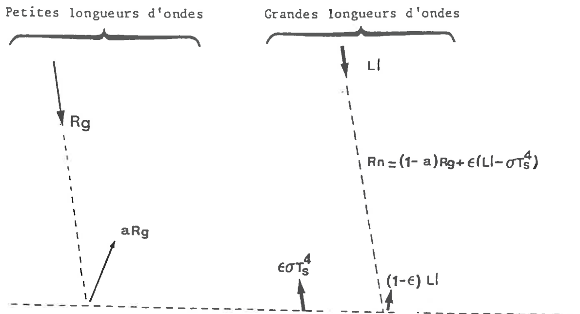
FIGURE I.3: Schéma du bilan radiatif
