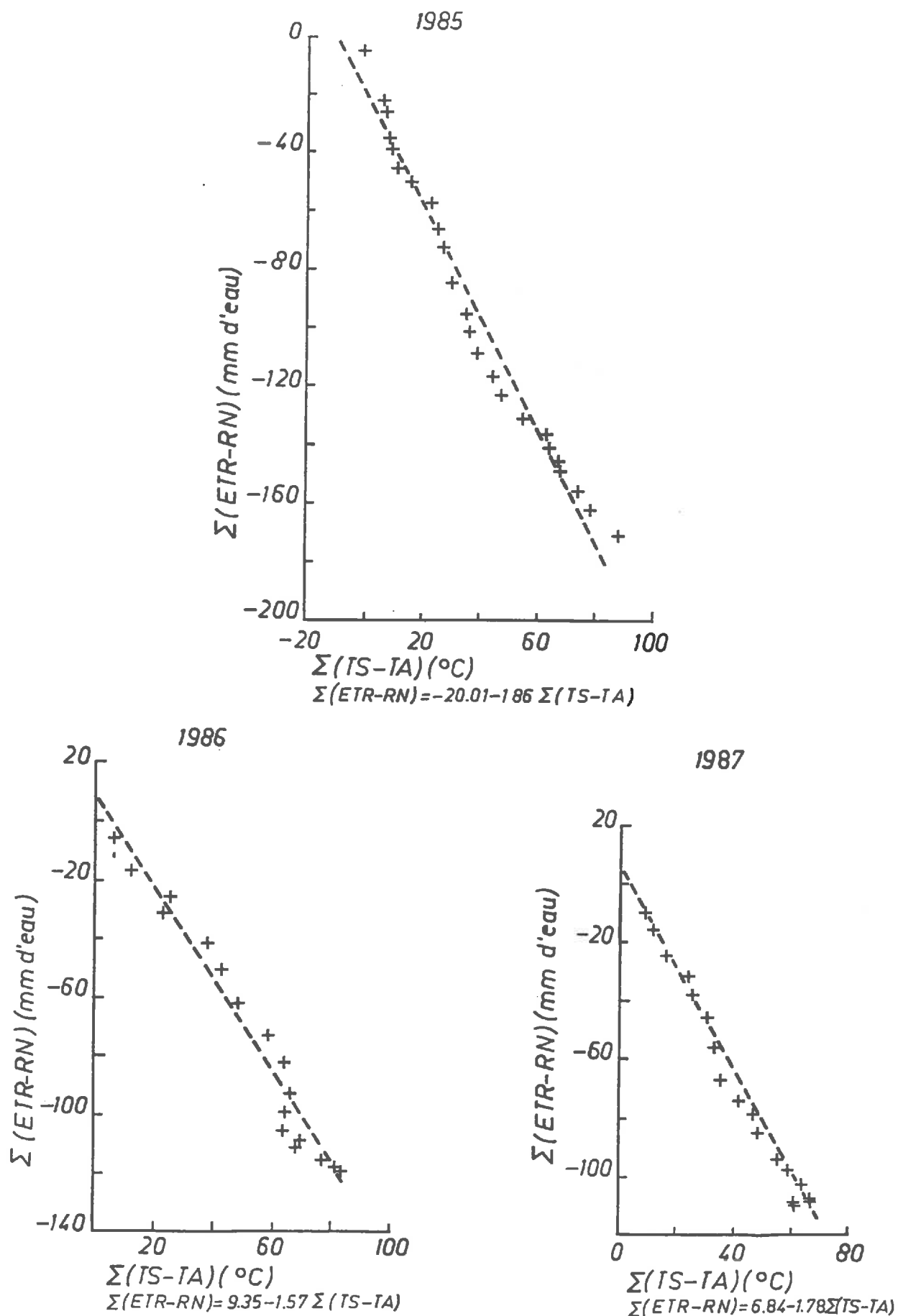
FIGURE V.12: Régressions linéaires obtenues à partir des valeurs de \Sigma(ETR-Rn) du modèle de CHOISNEL et de \Sigma(Ts-Ta) de METEOSAT: station de Mirecourt.
