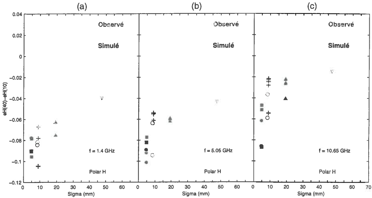
Figure E.3: évolutions expérimentales et modélisées de la variation angulaire de l'émissivité e(40 \text{ deg.}) - e(10 \text{ deg.}) en fonction de la moyenne des écart-type des hauteurs mesurés, en polarisation H, en conditions humides, à (a) 1.4 GHz, (b) 5.05 GHz, (c) 10.65 GHz.
