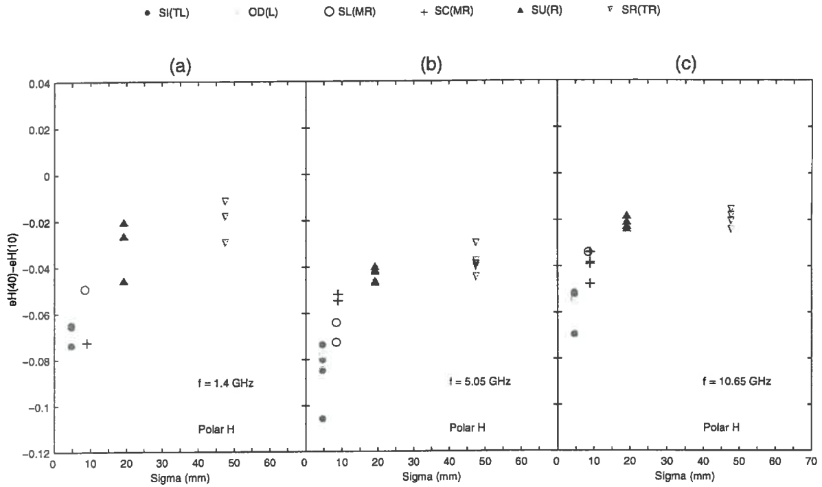
Figure 7.6: variations expérimentales de la différence angulaire de l'émissivité e(40 \text{ deg.}) - e(10 \text{ deg.}) en fonction de la moyenne des écart-type des hauteurs mesurés, en polarisation H , en conditions sèches, à (a) 1.4 GHz, (b) 5.05 GHz, (c) 10.65 GHz.
