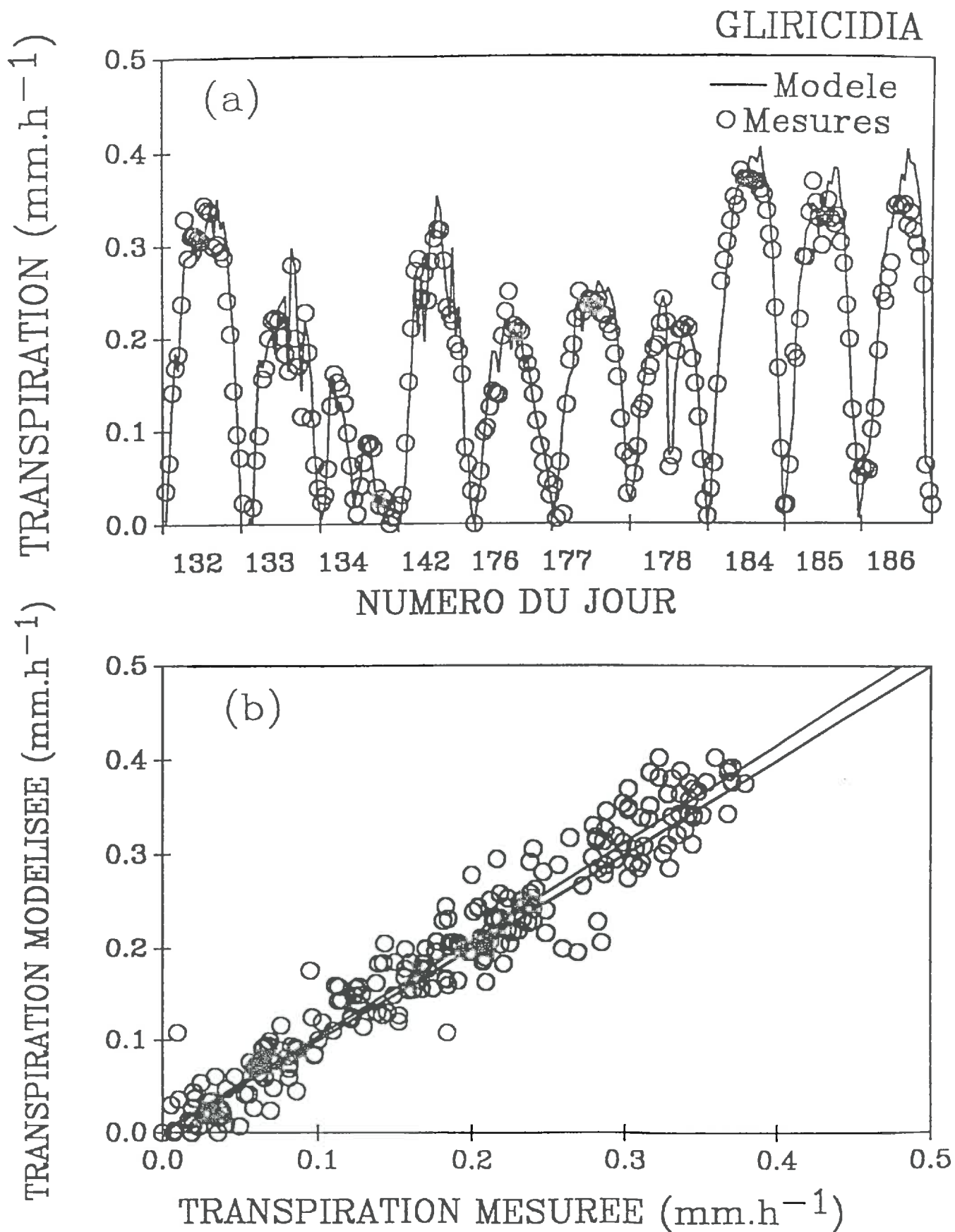
Figure IV.13. Comparaison entre la transpiration mesurée et celle modélisée pour l'arbust GLIRICIDIA (a) cinétique diurne (6h - 18h), au cours des dix jours de simulation et (b) regression.
