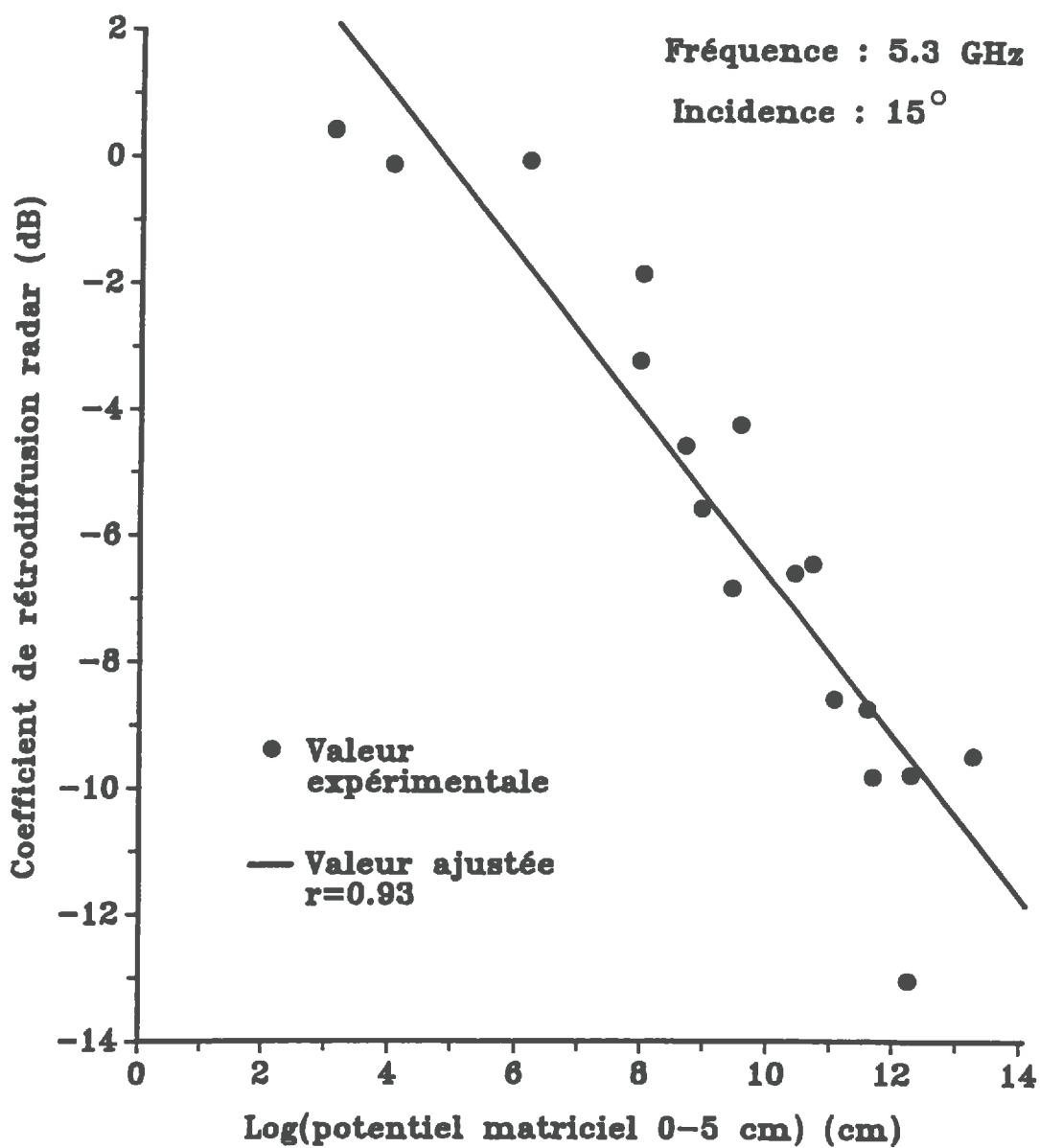
Figure 62 Relation entre le coefficient de rétrodiffusion radar et le potentiel matriciel du sol (polarisation HH)
