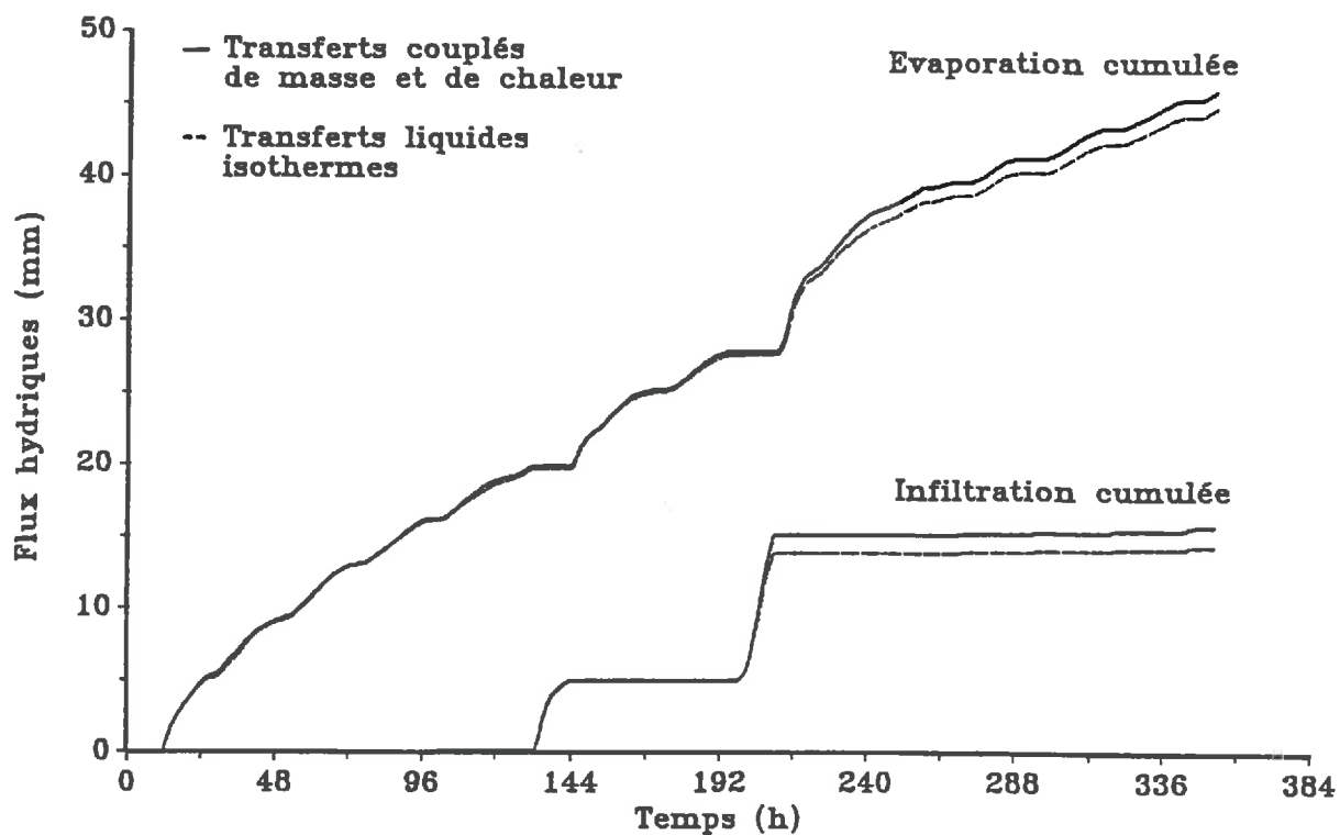
Figure 37 Comparaison de l'évaporation et de l'infiltration calculées entre le modèle de transferts couplés d'eau et de chaleur et le modèle de transferts en phase liquide en condition isotherme (simulation).
