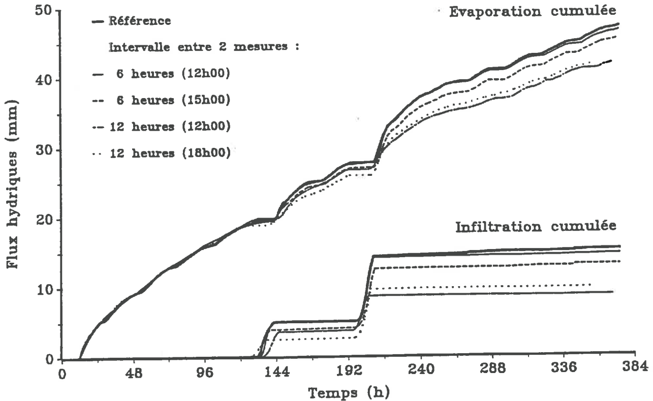
Figure 94a Evaporation et infiltration cumullées pour différentes mesures de teneur en eau de surface disponibles au cours du temps (Tab. 26) et modèle de référéncé.
