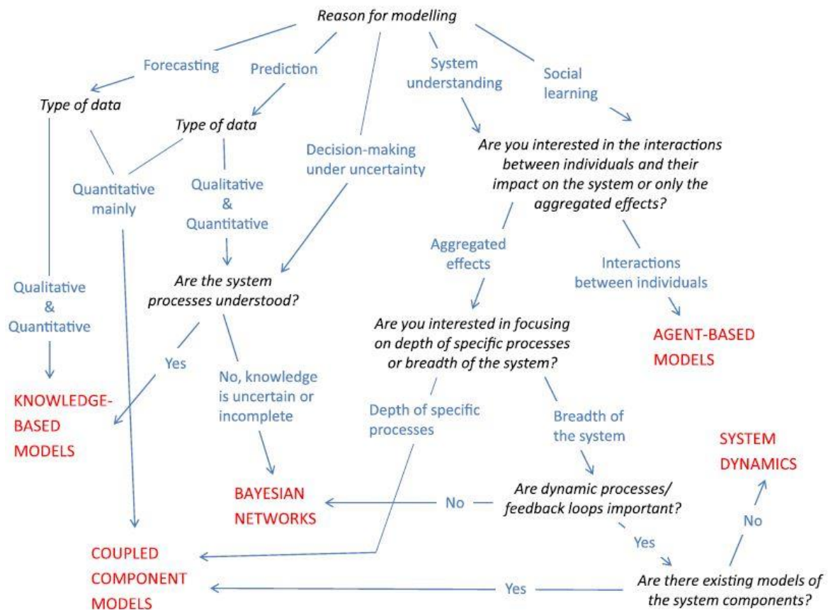
Figure 7. Arbre de décision pour le choix de la méthode de modélisation appropriée au problème (Kelly et al., 2013)
