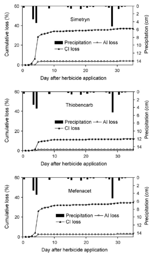
Figure 52. Pertes cumulées en pesticides (Simetryn, Thiobencarb et Mefenacet) selon la gestion hydraulique de l'irrigation en parcelles rizicoles expérimentales (site de Tsukuba, Watanabe et al. 2006).
