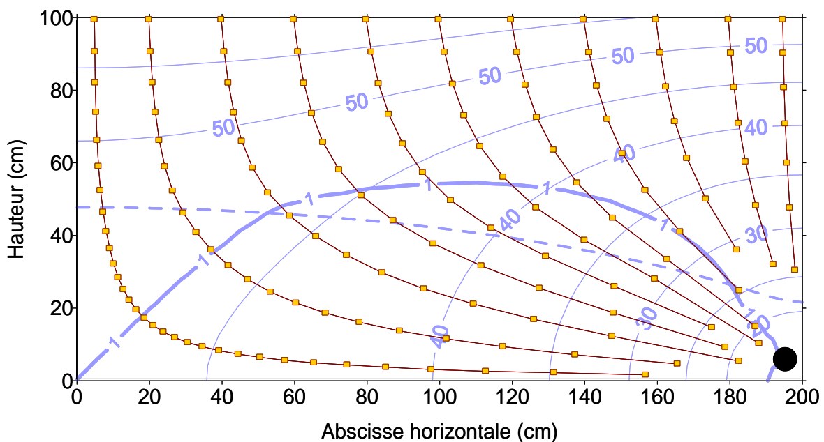
Figure 30. Trajectoires des particules appliquées en surface, à partir de données expérimentales acquises sur MASHYNS. En arrière plan sont figurés les courbes d'équipotentielle (charge hydraulique), les pointillés représentent la position de la nappe, chaque carré représente un pas de temps de 5h (Paris-Anguella, 2004)
