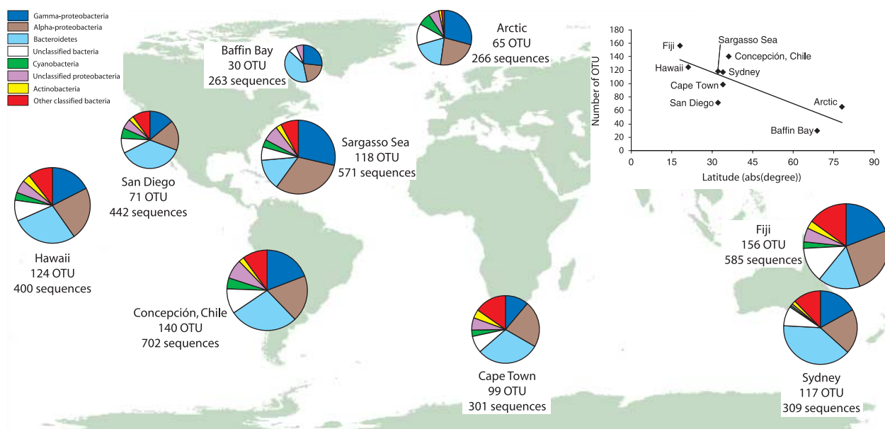
Fig. 4. Échantillonnage global de neuf communautés de bactérioplancton marin de surface (~5m) à l'échelle globale. La richesse locale en OTUs et le nombre de séquences obtenues par clonage sont indiqués en complément de la distribution des grandes classes taxonomiques échantillonnées (légende en haut à gauche). La taille de chaque camembert est proportionnelle à la richesse locale. La relation négative entre richesse et latitude (i.e. gradient latitudinal de richesse) est indiquée en haut à droite ( R^2=0.51 ; p<0.005 ) ; issu de Pommier, T. et al. , 2007.
