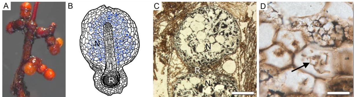
Fig. 58. Nodules mycorhiziens. (A) sur une racine de kauri actuel, (B) schéma d'une racine (R) portant un nodule (N) contenant des champignons (en bleu), (C) racine de conifère du Trias d'Antarctique portant deux nodules, (D) détail d'un nodule fossile contenant des hyphes de champignon (flèche). Echelles : C = 250 µm, D = 30 µm.
