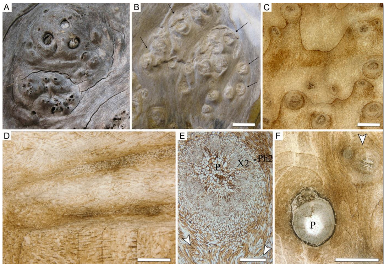
Fig. 51. Pousses épïcormiques (A) sur le tronc d'un érable actuel ayant perdu son écorce, (B-F) sur le tronc décortiqué d'une Glossoptéridale du Permien d'Antarctique : (B) vue externe, (C, D) sections montrant les traces vasculaires vues de face et longitudinalement, (E) détail d'une trace, (F) branche morte isolée au centre du tronc (noter la compartimentalisation indiquée par le tissu sombre autour de la branche). La perte/décomposition de cette branche pourrait avoir entraîné la formation des rameaux épïcormiques dans cette zone. Echelles : B = 5 mm, C, F = 2.5 mm, D = 2 mm, E = 500 \mu m.
