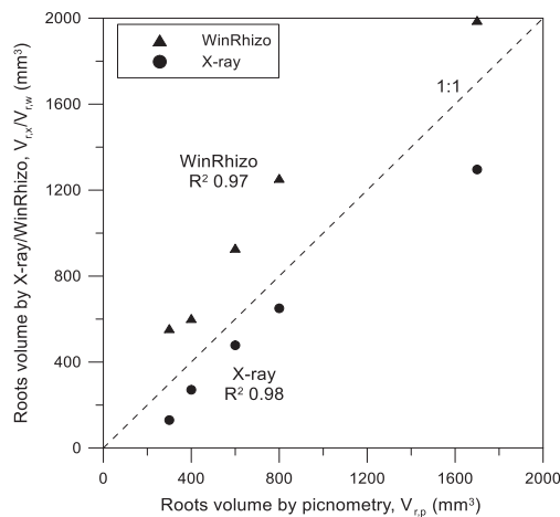
Figure 64 Comparaison des valeurs du volume des racines obtenues à partir de microtomographie rayon X, WinRhizo et picnométrie.
