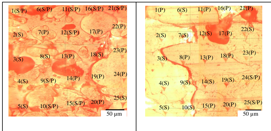
Figure Annexe-6.1. Images de microscopie optique des empreintes générées lors de l'indentation des composites de pois (S : amidon, P : protéine, F : phases de fibres, S/P : interphase amidon/protéine, S/F : interphase amidon/fibre et P/P : empreintes au contact entre les particules de protéines).
