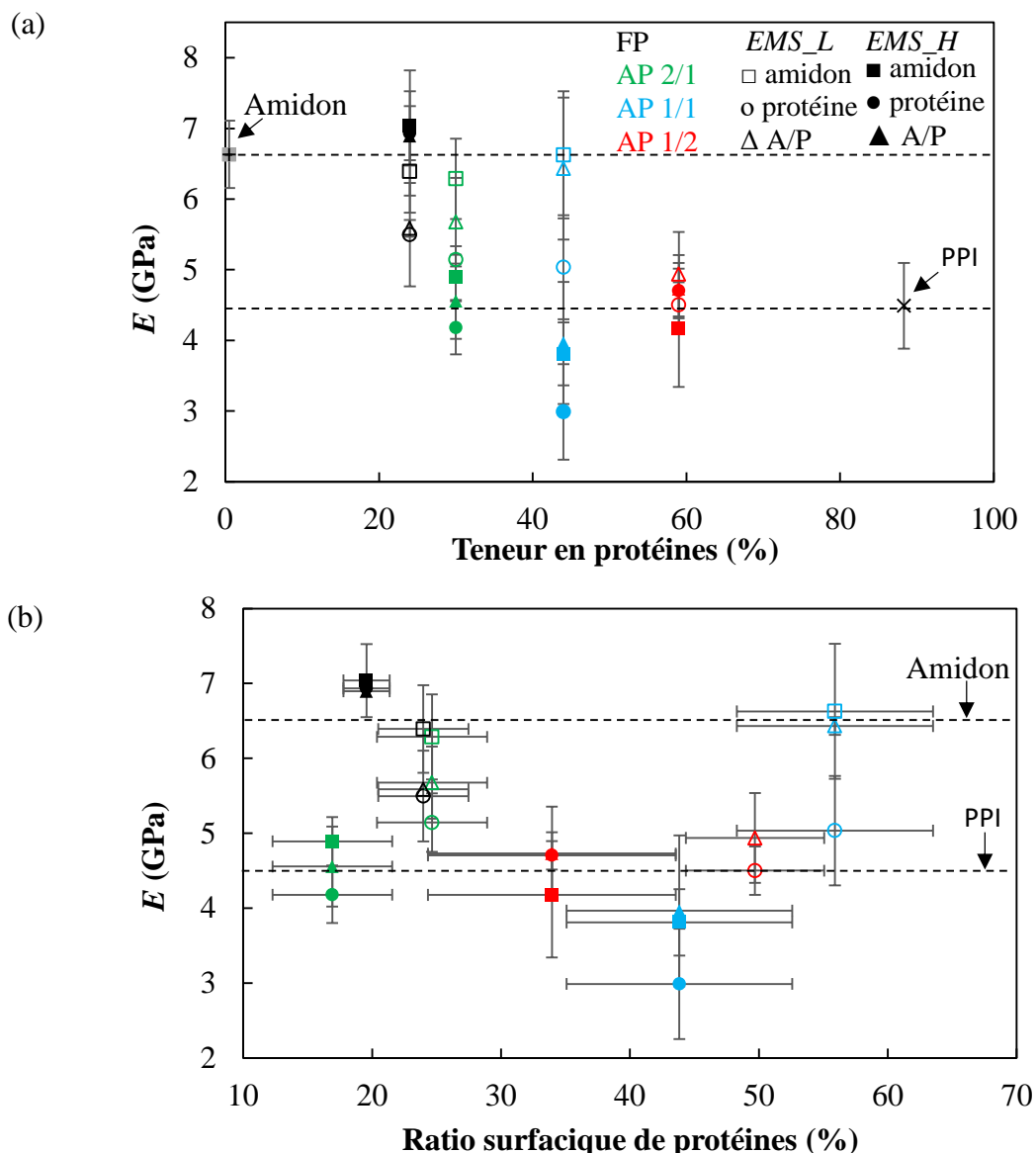
Figure 109. Variation du module de Young ( E ) des phases de l'amidon (□, ■) et de protéine (○, ●), et de l'interphase A/P (▲, △) avec (a) la teneur en protéines des composite et (b) le ratio surfacique de protéines déterminé par analyse des images MCBL pour les composites de farine de pois (●), mélanges AP2/1 (●), AP 1/1 (●) et AP 1/2 (●). Les symboles vides et pleins font référence aux échantillons extrudés à une EMS faible et élevée, respectivement. Les
