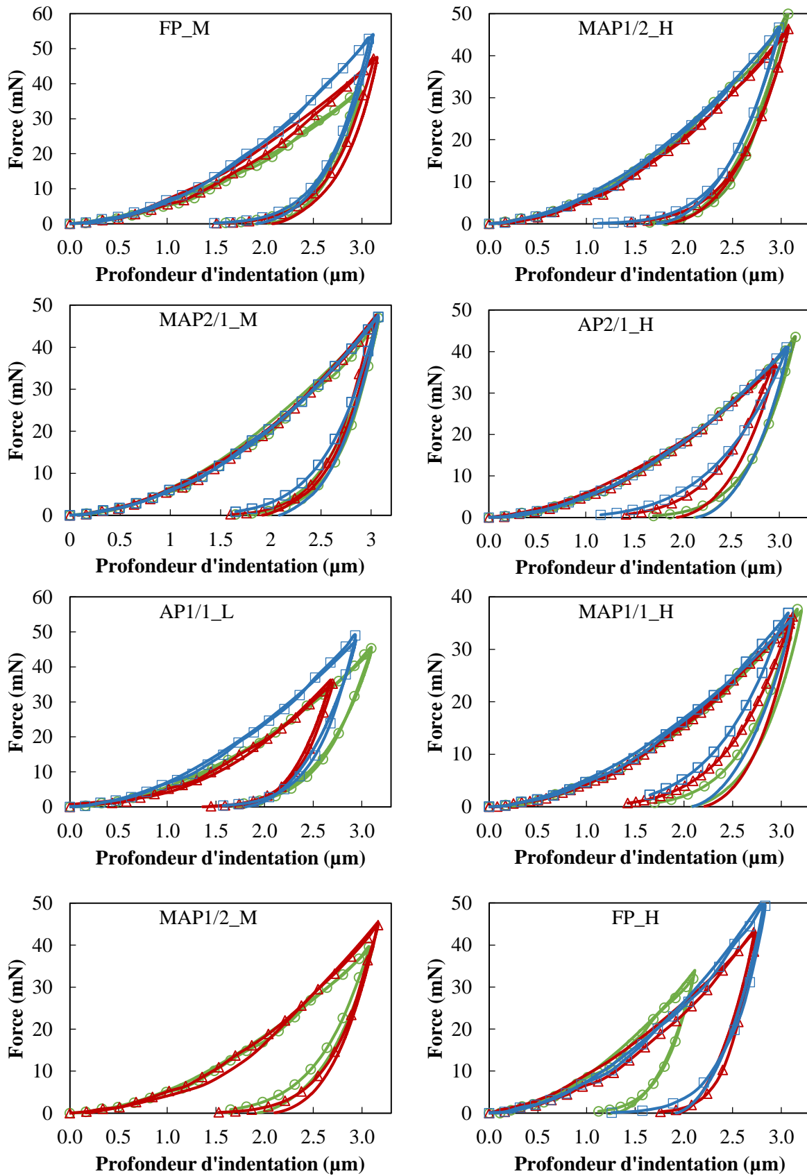
Figure 126. Comparaison des courbes d'indentation sur les phases d' amidon , protéine et l' interphase issues des essais expérimentaux (ligne continue) et de la simulation numérique (lignes avec symboles).
