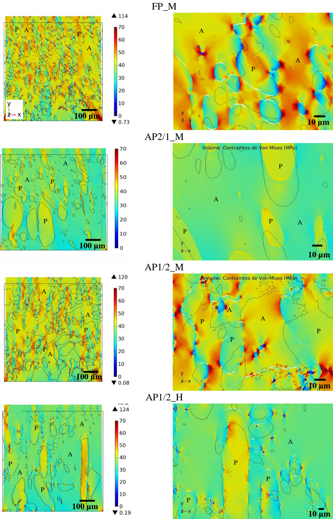
Figure 133. Distribution de la contrainte de Von Mises sur la microstructure (634 × 634 μm 2 ). Les images à droite focalisent sur une zone (~120 x 120 μm 2 ) de chaque microstructure de composite. Les tracés noirs correspondent au périmètre des particules protéiques à l'état initial
