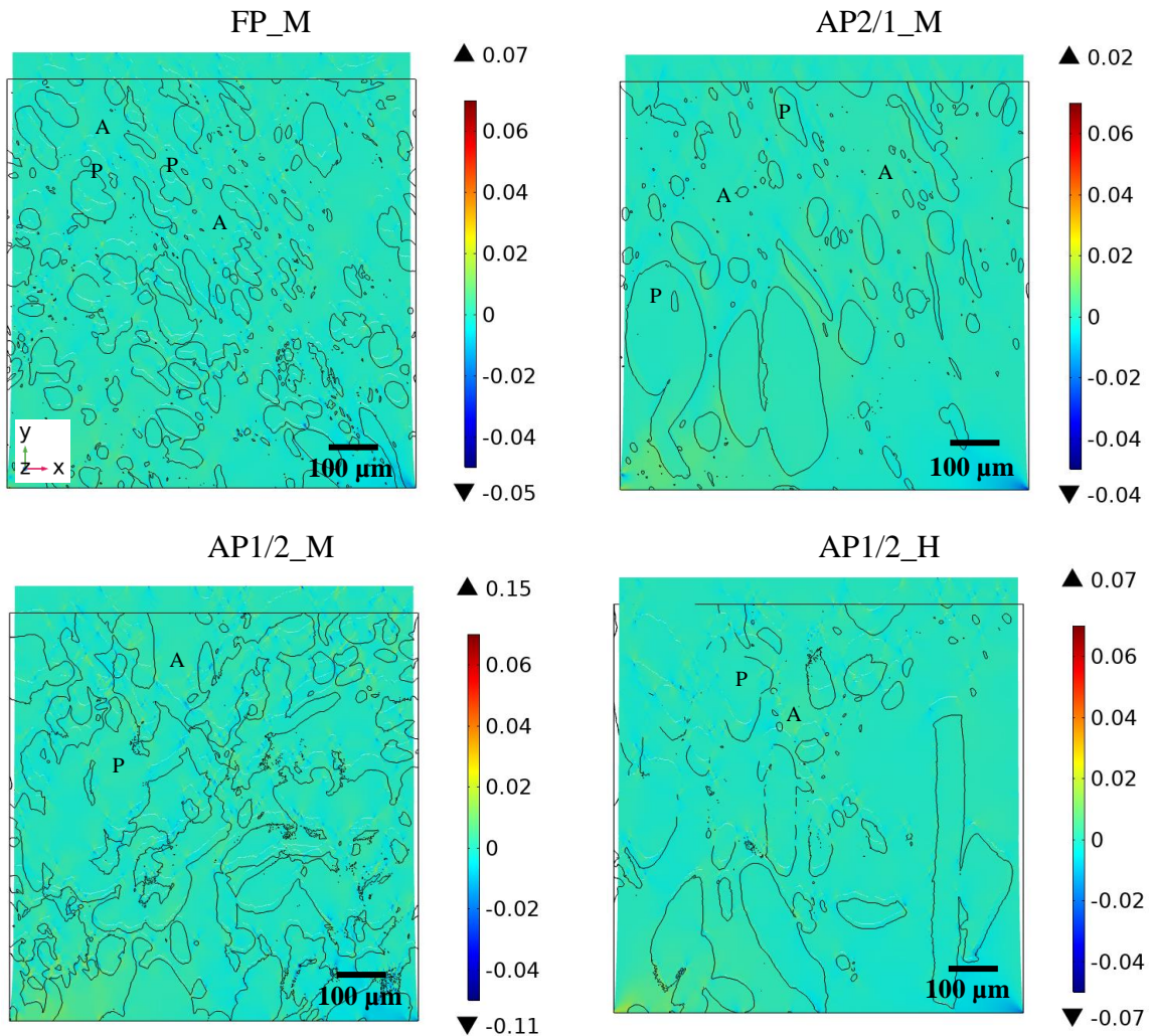
Figure 135. Distribution de la déformation locale en composante \varepsilon_{xy} (cisaillement) sur la microstructure ( 634 \times 634 \times 5 \mu\text{m}^3 ). Les tracés noirs correspondent au périmètre des particules protéiques à l'état initial avant la traction. L'espace blanc correspond à des vides à l'interface entre l'amidon et les protéines générés par la traction de la microstructure. P: Protéine, A: Amidon.
