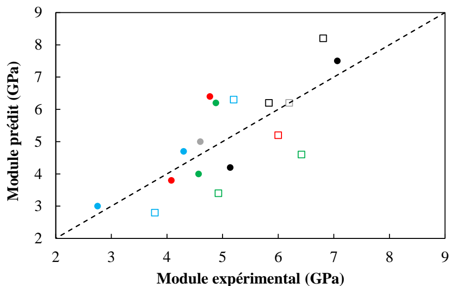
Figure 128. Comparaison de valeurs de module de Young ( E ) obtenues par le test de nanoindentation expérimental et par le calcul éléments finis pour les phases d'amidon ( \square ) et de protéines ( \bullet ) des composites de farine de pois, mélanges AP 2/1 ( \square, \bullet ), AP1/1( \square, \bullet ) et AP1/2 ( \square, \bullet ), ainsi que pour l'amidon thermomoulé ( \square ) et le PPI extrudé ( \bullet ).
