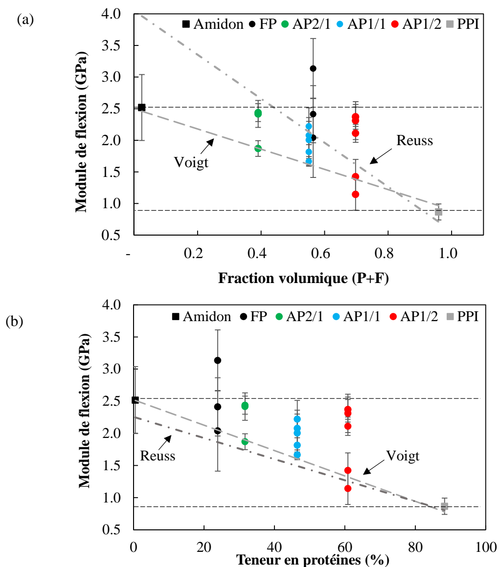
Figure 92. Variation de module de flexion avec (a) la fraction volumique de protéines et fibres (P+F), et (b) la teneur en protéines des matériaux. Les courbes pointillées correspondent à
