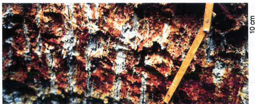
Photo 5 : Planosol (savane de Corossony). Coupe verticale entre 140 et 170 cm de profondeur. Vue de détail de pores tubulaires verticaux d'origine racinaire à gaine bleutée traversant l'horizon sablo-argileux rougeâtre B G o/r .
