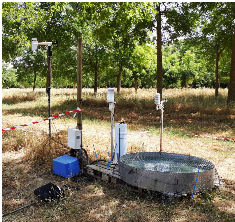
FIGURE 19 Bac d'évaporation de classe A installé en AF (bloc B) pendant la période estivale.
