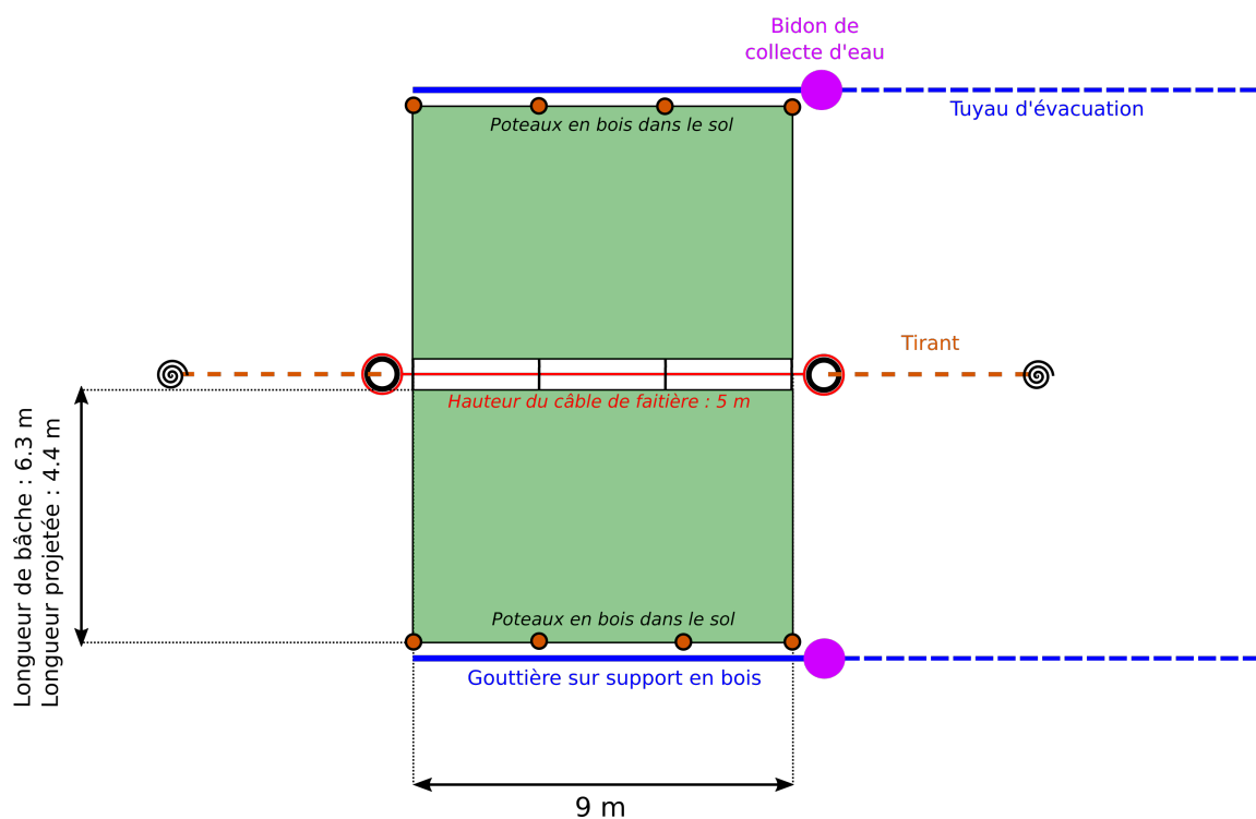
FIGURE C.3 Schéma global du dispositif de grande envergure en témoin agricole
