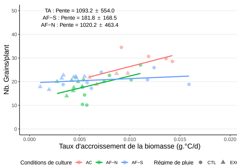
FIGURE IV.6 Régression entre le nombre de grain final par plante et le taux d'accroissement de biomasse (entre le début de la floraison et le stade limite de fin d'avortement) en fonction des conditions de culture.
