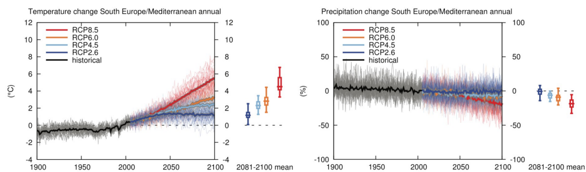
FIGURE 5 Projections climatiques établies du changement de la température et des précipitations moyennes annuelles en région Méditerranéenne selon le 5 ème rapport du GIEC (IPCC, 2013). Des projections spatialisées et à l'échelle saisonnière sont disponibles en Appendice A .
