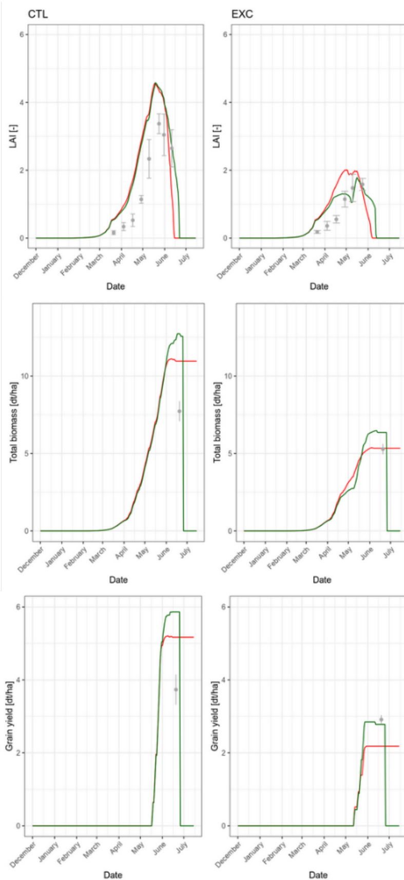
FIGURE F.2 Comparaison de la dynamique de LAI du pois d'hiver pour des scènes "identiques" entre Hi-sAFé 4.1 et STICS standalone (8.5) selon les deux régimes de pluie. Les observations sont présentées en gris, les simulations Hi-sAFé en vert foncé et les simulations STICS en rouge.
