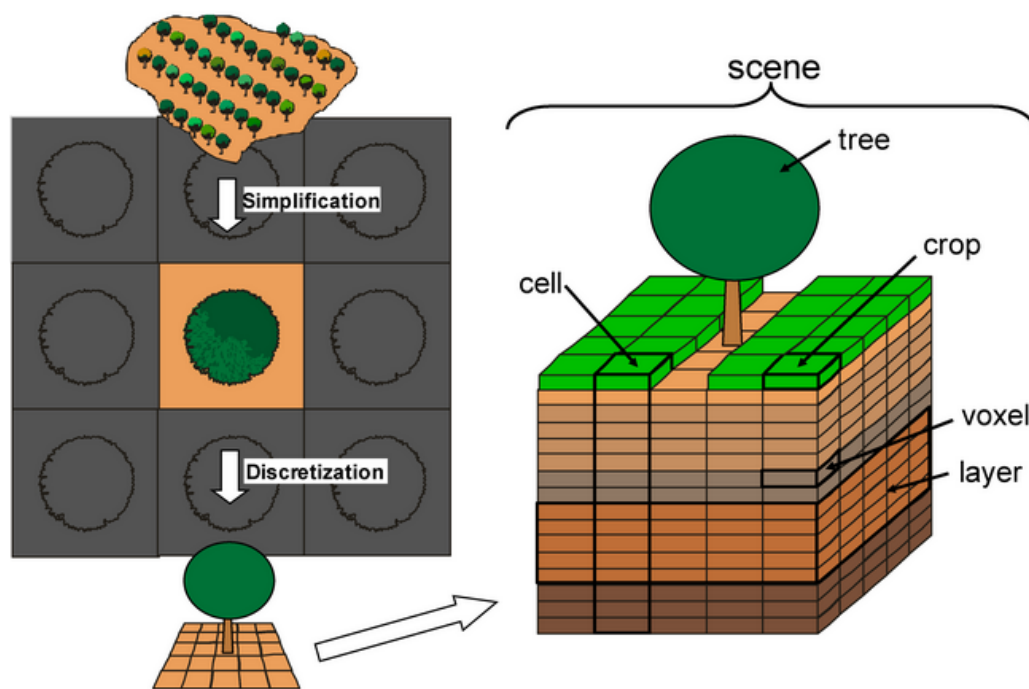
FIGURE IV.5 Scène virtuelle Hi-sAFé et ses différents éléments. Figure tirée de Dupraz (2019)
