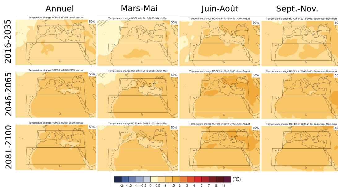
FIGURE A.2 Anomalie médiane des températures à l'échelle de l'année et des saisons pour le bassin Méditerranéen selon le scénario RCP2.6 . Les données sont exprimées relativement à la période 1986-2005. Graphique établi à partir du 5 ème rapport du GIEC (IPCC, 2013)
