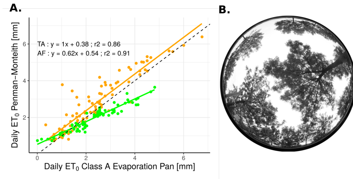
FIGURE IV.7 Comparaison de l'ETP0 journalière estimée selon les mesures à partir du bac d'évaporation (axe des abscisses) et selon les données météorologiques (axe des ordonnées). La relation est évaluée en TA (points oranges) et en AF (points verts).
