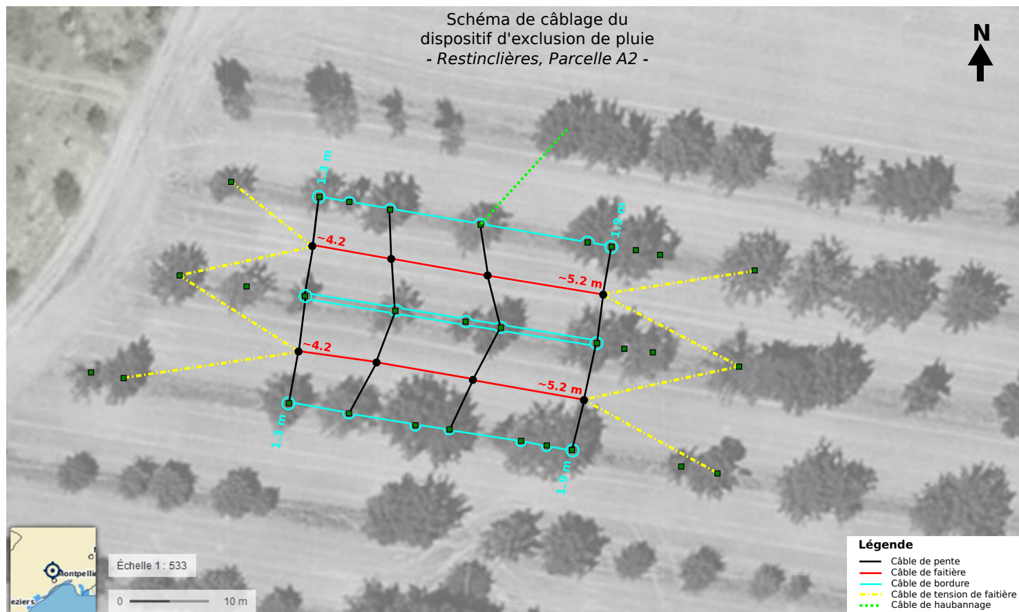
FIGURE C.4 Schéma global de l'implantation des câbles de structure du dispositif de grande envergure en agroforesterie
