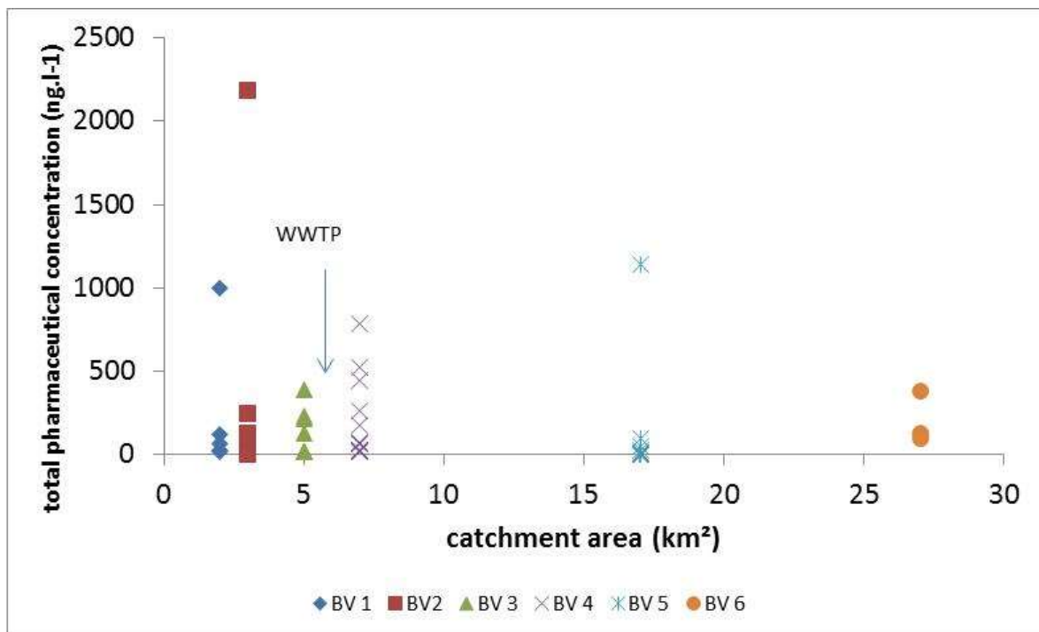
Figure 31 : Localisation des points de suivi et de la station d'épuration (haut), et variabilité spatiale des concentrations totales en RM en fonction de l'aire drainée bas).
