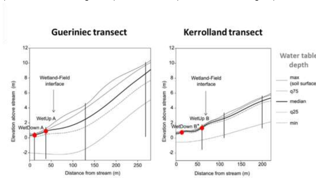
Figure 18: topographie des transects piézométriques de Guerinieci et Kerrolland et profondeur de la nappe (min, max, médiane) mesurée sur 10 ans.
