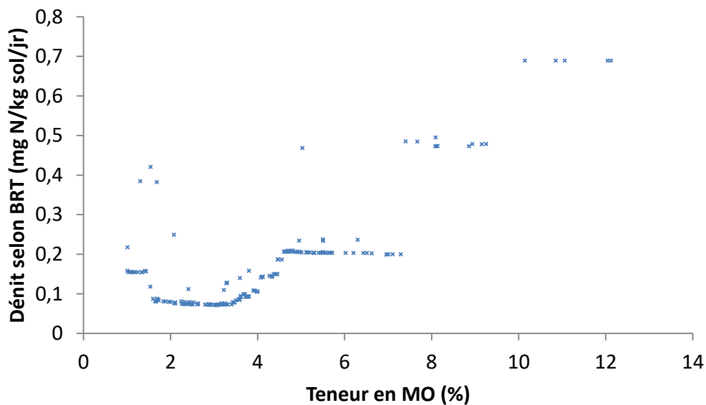
Figure 38 : photos de profil de sols, Epaisseurs et teneurs en MO des 270 horizons organominéraux de sol de zones humides (haut) et dénitrification estimée par le modèle BRT (Oehler et al., 2010) sur les 191 horizons dans le domaine de validité du modèle
