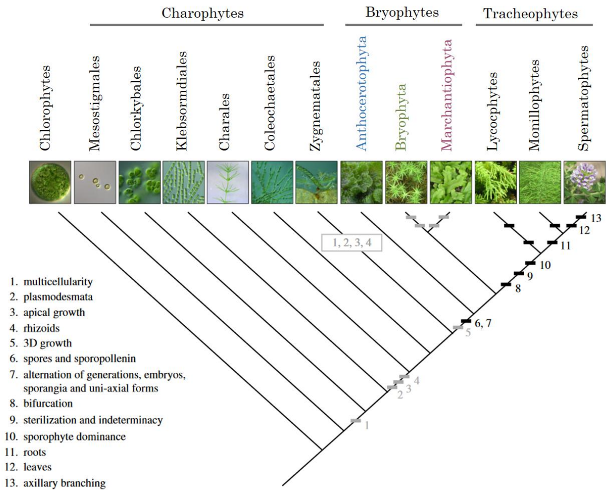
Figure 7 – Arbre phylogénétique présentant les innovations pour les gamétophytes (barres grises) et pour les sporophytes (barres noires). Adapté de Harrison, 2017.
