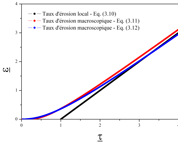
Fig. 3.9 – Loi d'érosion locale (Eq. 3.10) et lois d'érosion macroscopique, sans distribution statistique sur la contrainte critique \tau_c (Eq. 3.11) et avec une distribution statistique très large où \sigma_c = \langle \tau_c \rangle (Eq. 3.12). Toutes ces lois sont tracées en coordonnées sans dimension : \underline{\epsilon} en fonction de \underline{\tau} .
