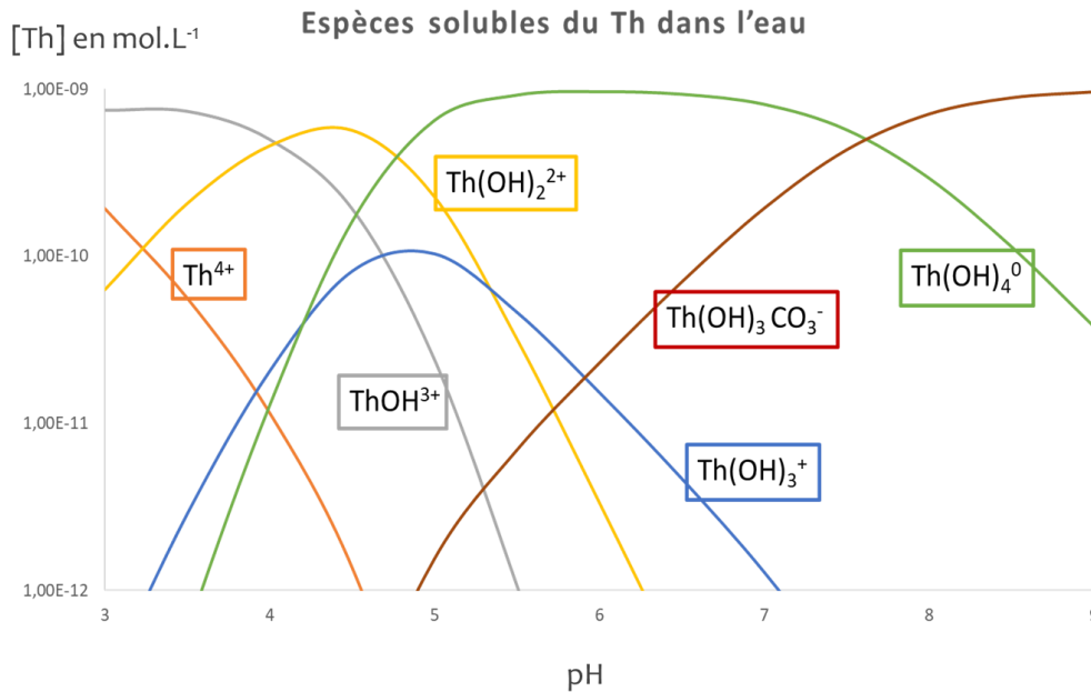
Figure 2.3. Spéciation du thorium concentré à 1 nM dans l'eau en fonction du pH modélisé à l'aide du logiciel WHAM et des données thermodynamiques issues de la base de données Nagra/PSI 01/01 [25]
