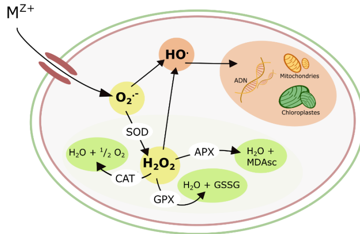
Figure 1.4. Schéma général des mécanismes de génération du stress oxydatif par le cation métallique M^{Z+} et ses conséquences dans les cellules algales suite à une internalisation (adapté de Pinto et al., 2003). Les abréviations : superoxyde dismutase (SOD), catalase (CAT), ascorbate peroxydase (APX), glutathion peroxydase (GPX), molécules de glutathion liées par une liaison disulfide (GSSG), monodehydroascorbate (MDA sc )
