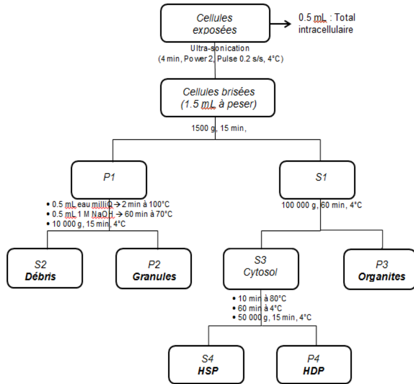
Figure 2.1. Représentation de la méthode de fractionnement subcellulaire appliquée à l'algue C. reinhardtii traduit de Lavoie et al. (2009) [20] et les différentes fractions obtenues : débris, granules, organites, protéines stables à la chaleur (HSP) et protéines instables à la chaleur (HDP). Les abréviations P et S signifiant culot ( pellet ) et surnageant respectivement.
