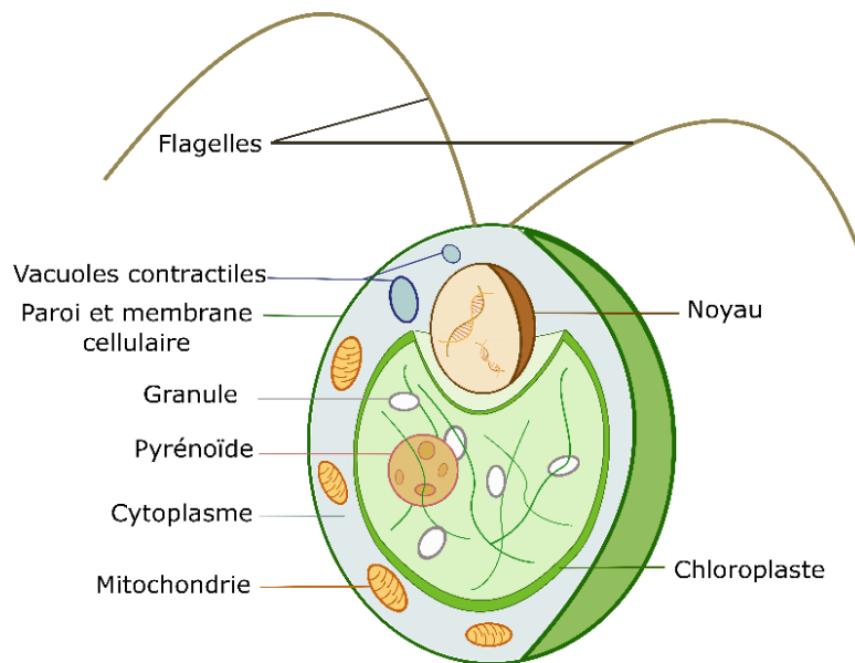
Figure 1.6. Représentation schématique de Chlamydomonas reinhardtii
