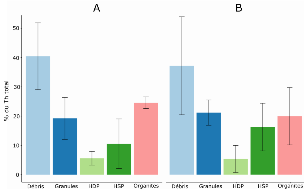
Figure 2.5. Répartition subcellulaire du Th chez l'algue verte Chlamydomonas reinhardtii (CR) après 1 h d'exposition en pourcentage de la somme des concentrations en Th mesurées dans les fractions. A. Conditions exposées à 1 nM de Th, les valeurs représentées sont les moyennes des trois répliques des trois expériences (n = 9). B. Conditions témoins les valeurs représentées sont les moyennes des échantillons des trois expériences (n = 3). Les barres d'erreurs correspondent aux écarts-types.
