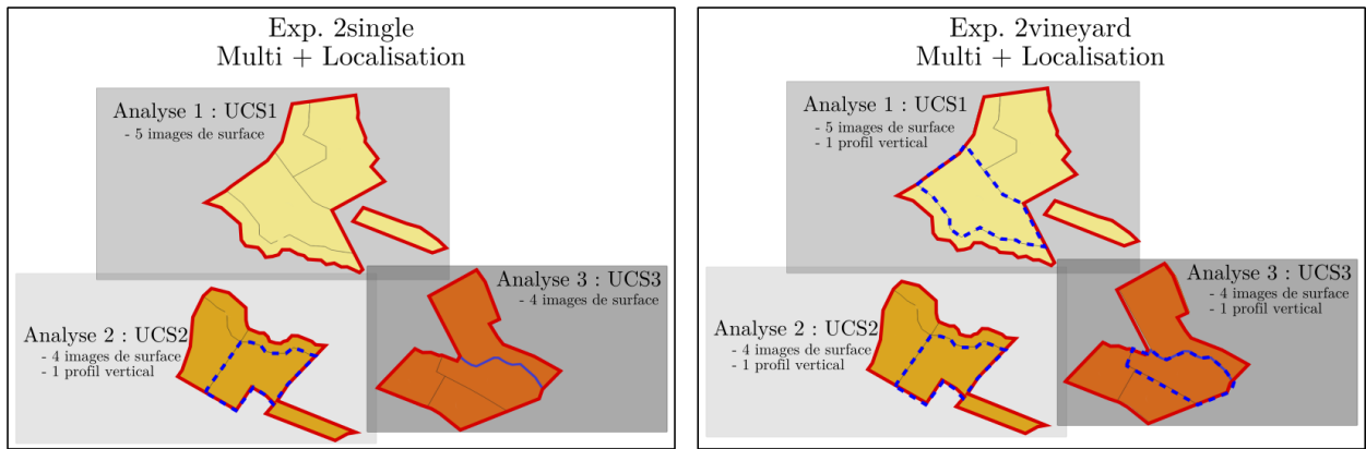
Figure 8.4 – Découpage de l'analyse mis en œuvre avec la localisation par domaines dans les expériences 2single/Multi et 2vineyard/Multi. Les UH entourées en bleu sont celles où l'on dispose de profils verticaux.
