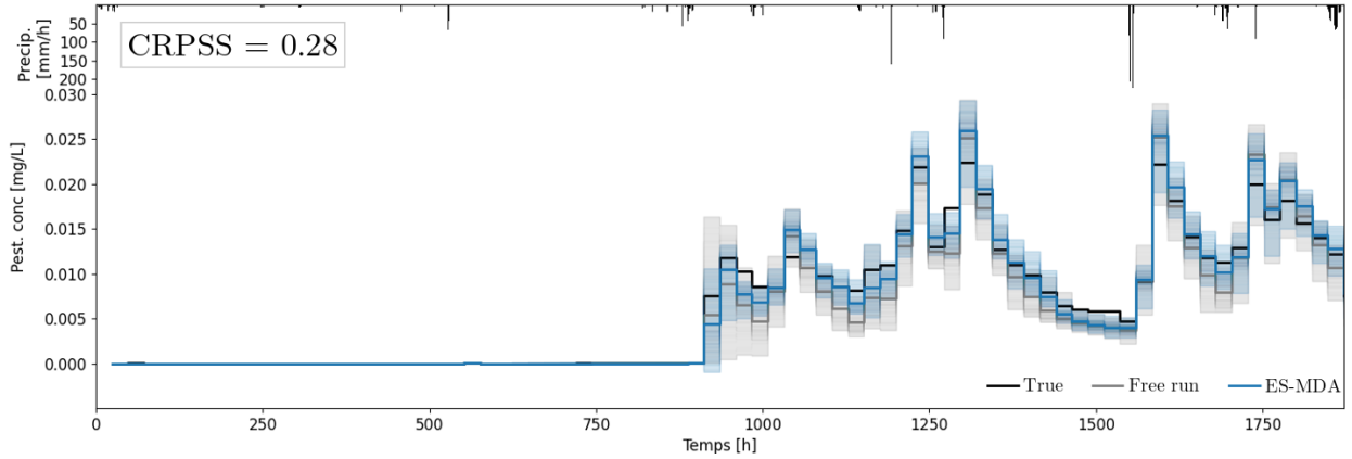
Figure 8.7 – Comparaison des trajectoires de concentration journalière moyenne à l’exutoire de la référence (“True”, noir), de l’ensemble non assimilé (“Free run”, gris) et de l’ensemble analysé (bleu) (Expérience 3hydro).
