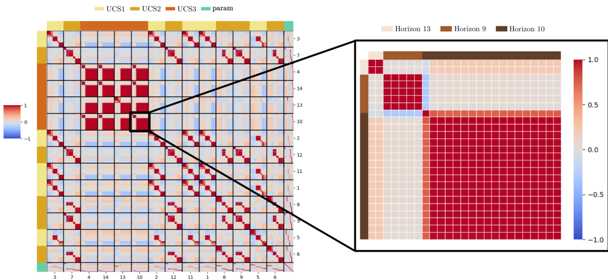
Figure 7.11 – Gauche : matrice de corrélation de l'ensemble après 144 h de simulation pour le free run sur l'ensemble des UH. Les lignes noires horizontales et verticales délimitent les cellules numériques d'une même UH. Les couleurs en haut et à gauche indiquent le type de sol de chaque UH alors que les numéros en bas et à droite indiquent les indices des UH. Droite : extrait de la matrice de corrélation correspondant à l'UH10. Chaque pixel délimite une cellule numérique du profil vertical de l'UH10. Les couleurs en haut et à gauche indiquent l'horizon de sol auquel appartient chaque cellule numérique.
