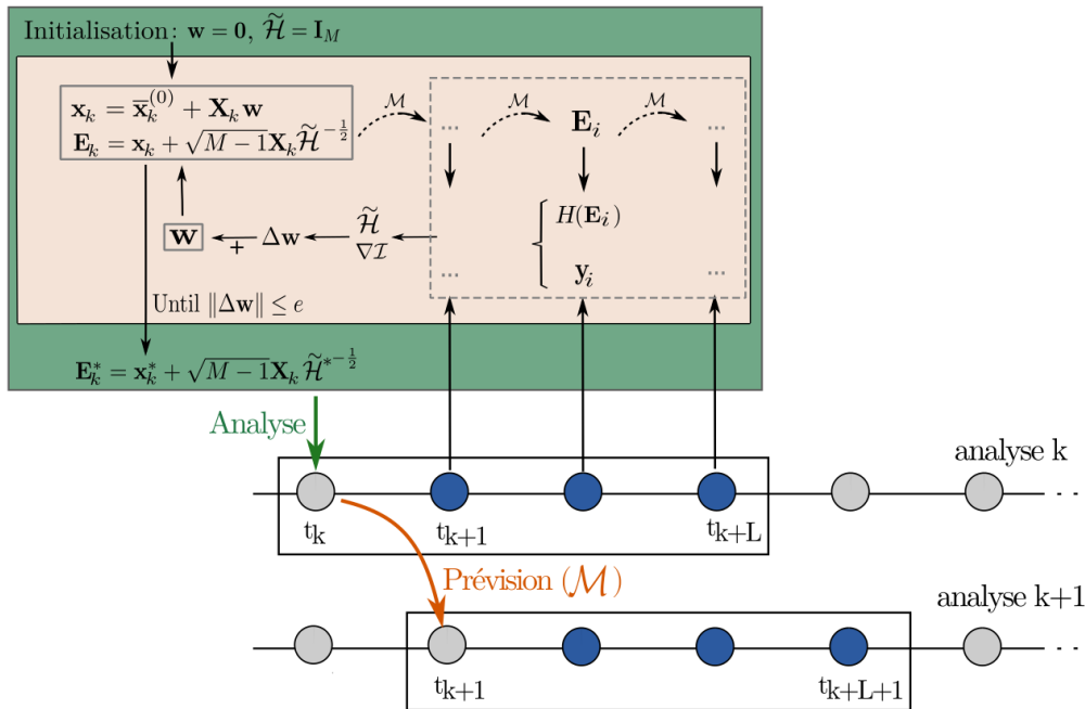
Figure 6.6 – Détails d'un cycle d'assimilation effectué par l'iEnKS ( \Delta \mathbf{w} désigne l'incrément \mathbf{w}_{(j+1)} - \mathbf{w}_{(j)} ). Dans cet exemple, L=3 . Les points bleus schématisent les observations utilisées pendant le cycle d'assimilation courant alors que les cercles gris illustrent les observations disponibles mais non utilisées.
