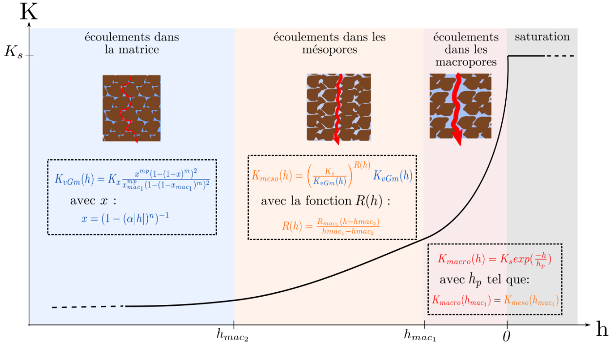
Figure 2.3 – Description de la courbe de conductivité utilisée dans PESHMELBA pour la résolution de l'équation de Richards selon la formulation de SCHAAP et VAN GENUCHTEN (2006).
