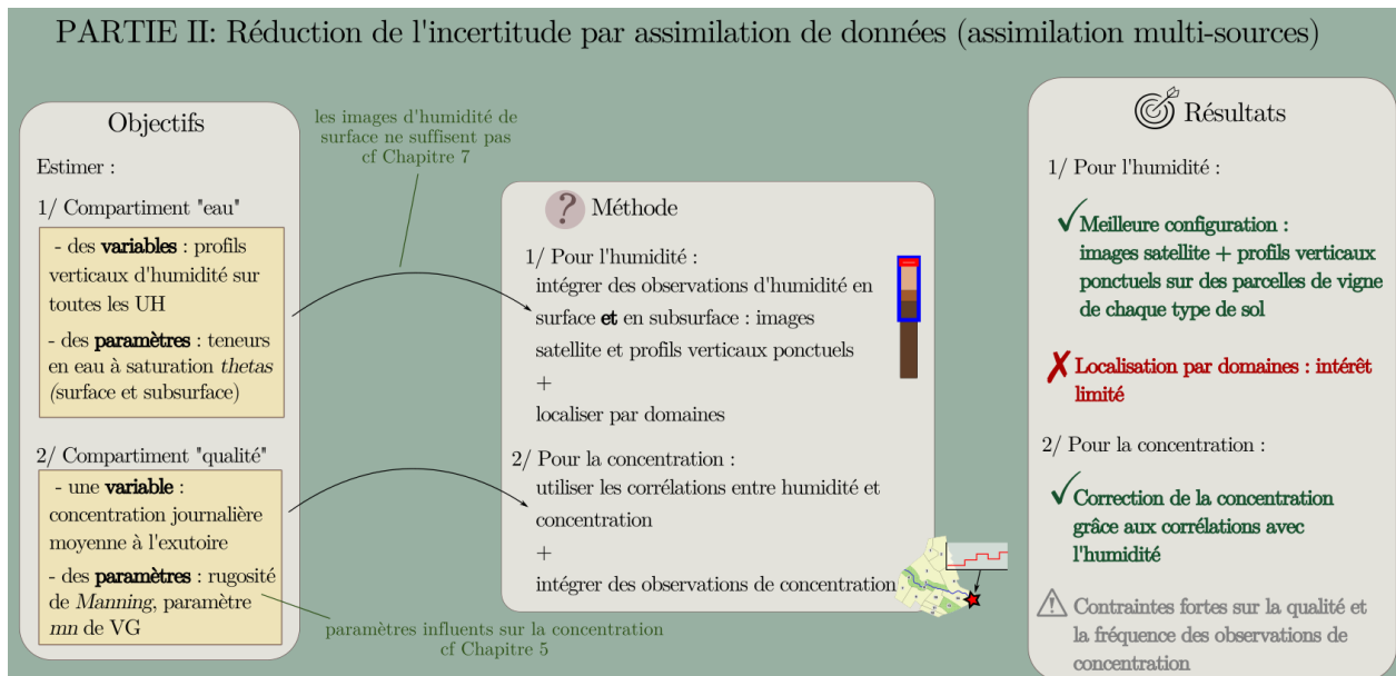
Figure 8.9 – Résumé visuel du chapitre 8 : objectifs de départ, outils utilisés et principaux résultats obtenus pour l'assimilation multi-sources.
