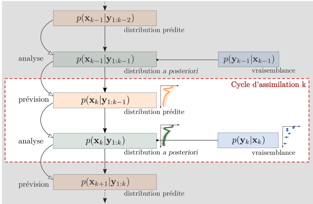
Figure 6.3 – Diagramme du filtrage séquentiel bayésien. Chaque cycle d’assimilation comprend une étape de prévision et une étape d’analyse.
