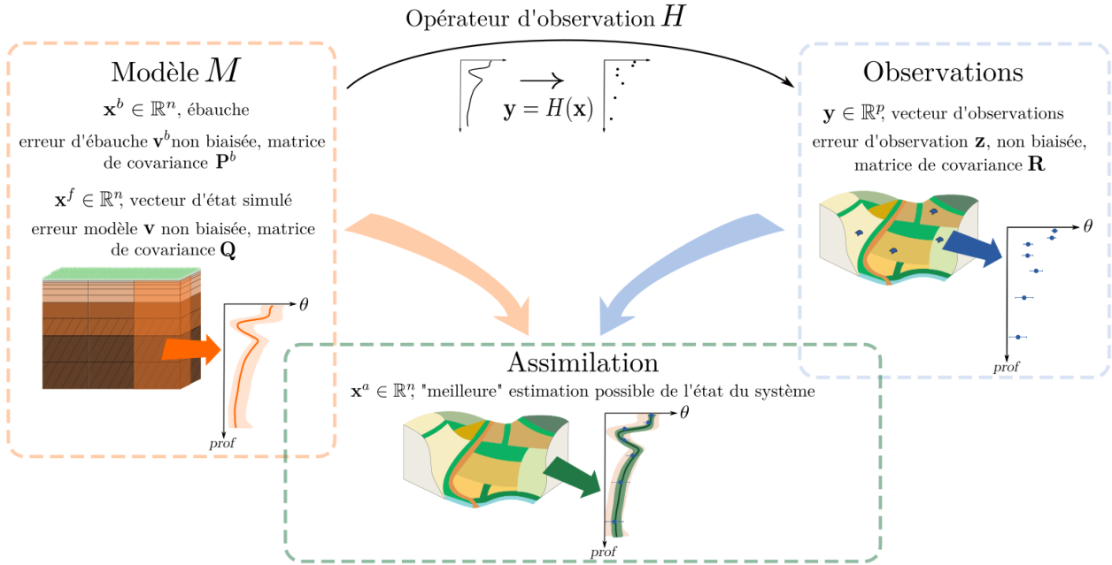
Figure 6.1 – Principe de l’assimilation de données, ingrédients et notations utilisés illustrés sur un exemple d’estimation de profils verticaux d’humidité.
