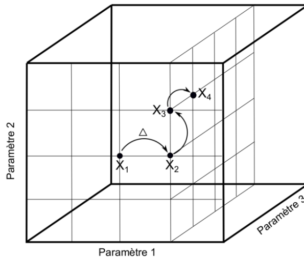
Figure 3.3 – Exemple de trajectoire de Morris échantillonnée dans un espace à trois dimensions avec 5 niveaux et un pas de discrétisation \Delta = 0.25 (tiré de DAIRON 2015).
